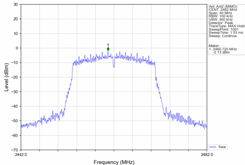
802.11n(HT20)_HCH_2462MHz_Ant2 (MIMO)_NTNV
