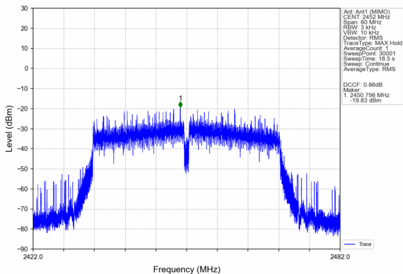
802.11n(HT40)_HCH_2452MHz_Ant1 (MIMO)_NTNV
