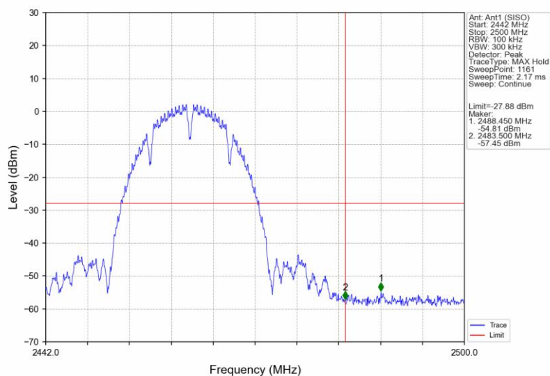
802.11b_HCH_2462MHz_Ant1 (SISO)_NTNV
