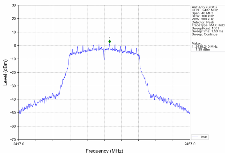
802.11g_MCH_2437MHz_Ant2 (SISO)_NTNV
