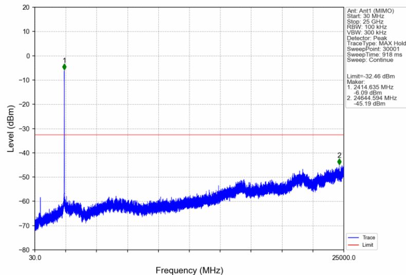
802.11n(HT20)_LCH_2412MHz_Ant1 (MIMO)_NTNV
