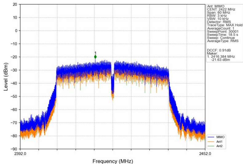
802.11n(HT40)_LCH_2422MHz_MIMO_NTNV
