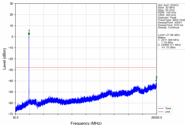
802.11b_LCH_2412MHz_Ant1 (SISO)_NTNV
