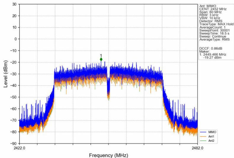
802.11n(HT40)_HCH_2452MHz_MIMO_NTNV
