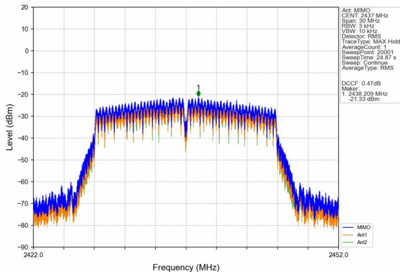
802.11n(HT20)_MCH_2437MHz_MIMO_NTNV
