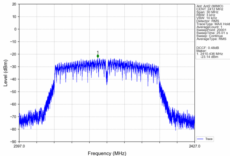
802.11n(HT20)_LCH_2412MHz_Ant2 (MIMO)_NTNW
