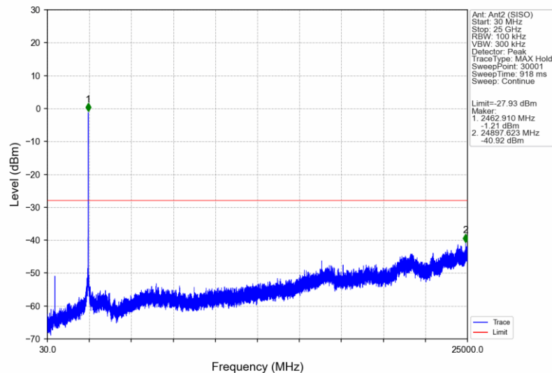
802.11g_HCH_2462MHz_Ant2 (SISO)_NTNV
