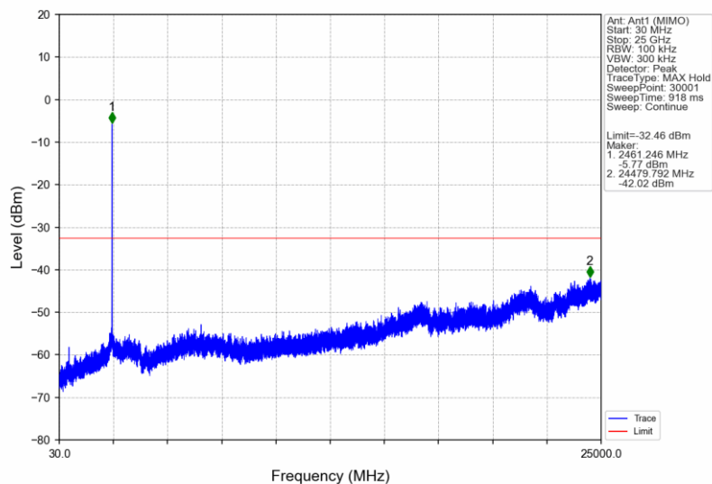
802.11n(HT20)_HCH_2462MHz_Ant1 (MIMO)_NTNV
