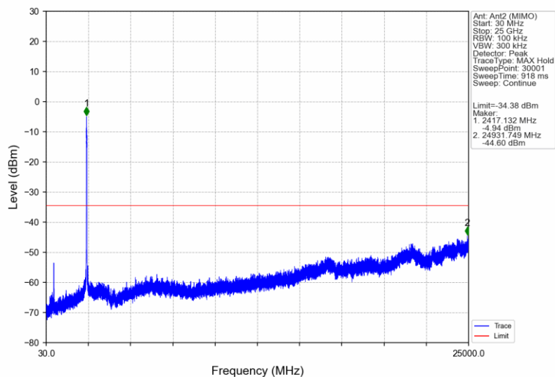
802.11n(HT40)_LCH_2422MHz_Ant2 (MIMO)_NTNV
