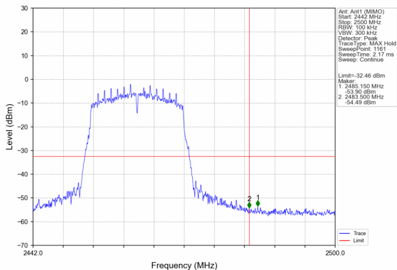
802.11n(HT20)_HCH_2462MHz_Ant1 (MIMO)_NTNV
