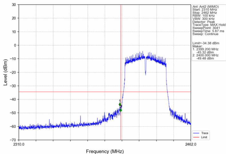
802.11n(HT40)_LCH_2422MHz_Ant2 (MIMO)_NTNV
