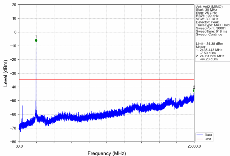
802.11n(HT40)_MCH_2437MHz_Ant2 (MIMO)_NTNV
