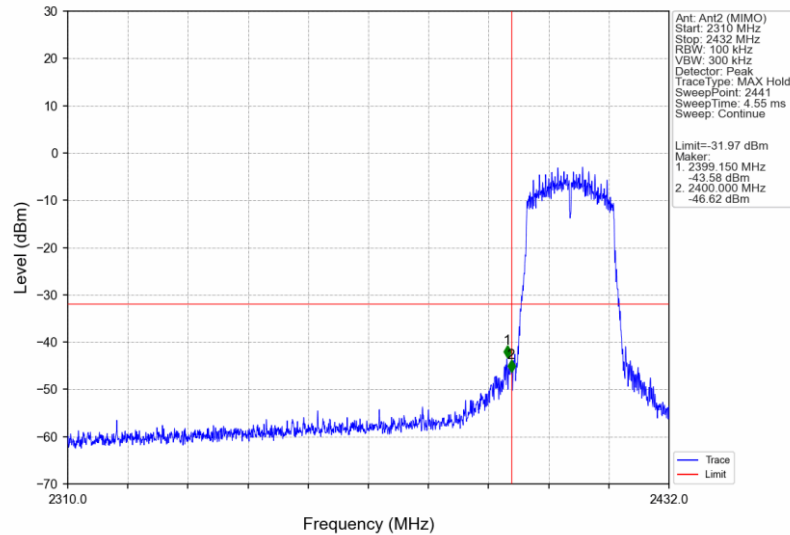
802.11n(HT20)_LCH_2412MHz_Ant2 (MIMO)_NTNV
