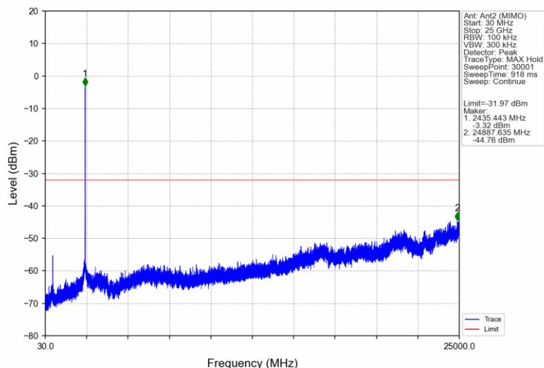
802.11n(HT20)_MCH_2437MHz_Ant2 (MIMO)_NTNV
