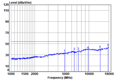
11n_HT(20M)_TX_CH_06_Horizontal-Avg
