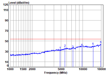
11n_HT(20M)_TX_CH_06_Vertical-Avg
