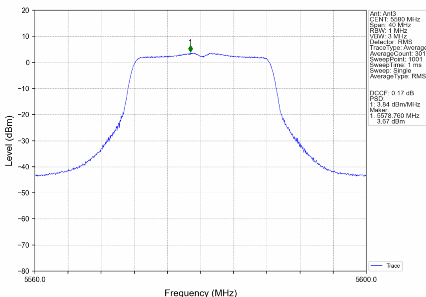
802.11a_MCH_5580MHz_Ant3_NTNV
