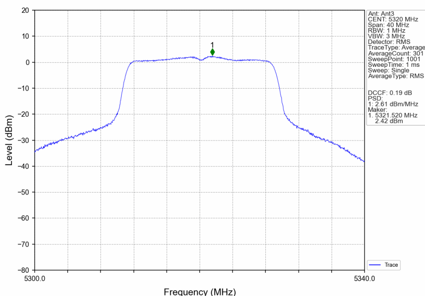
802.11n(HT20)_HCH_5320MHz_Ant3_NTNV
