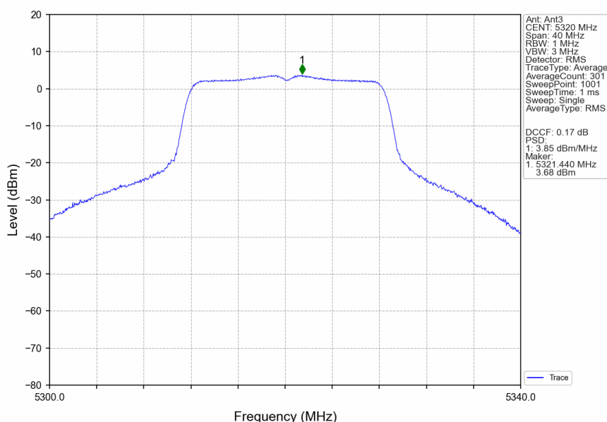
802.11a_HCH_5320MHz_Ant3_NTNV
