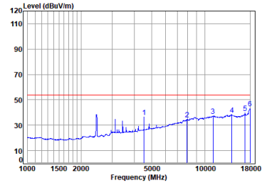
11ax_40M_TX_CH_09_Horizontal-Avg
