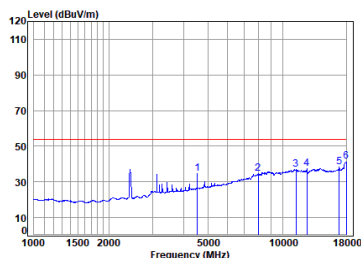
11ax_40M_TX_CH_06_Vertical-Avg
