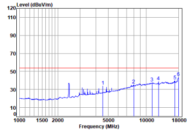
11ax_40M_TX_CH_09_Vertical-Avg
