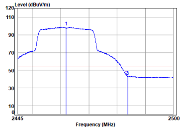
11ax_20M_TX_CH_11_Vertical-Avg
