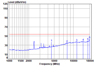
11ax_40M_TX_CH_03_Horizontal-Avg
