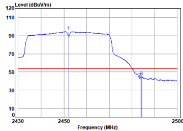
11n_HT(40M)_TX_CH_09_Vertical-Avg
