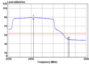
11n_HT(40M)_TX_CH_09_Horizontal-Avg
