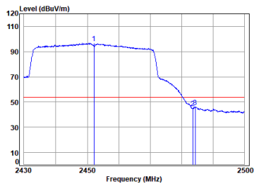
11ax_40M_TX_CH_09_Vertical-Avg
