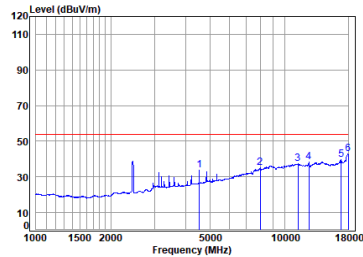
11n_HT(40M)_TX_CH_09_Vertical-Avg
