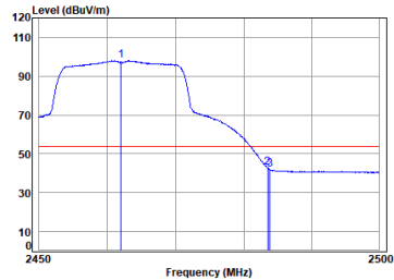
11n_HT(20M)_TX_CH_11_Vertical-Avg
