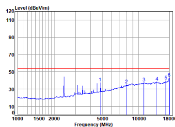
11b_TX_CH_01_Horizontal-Avg
