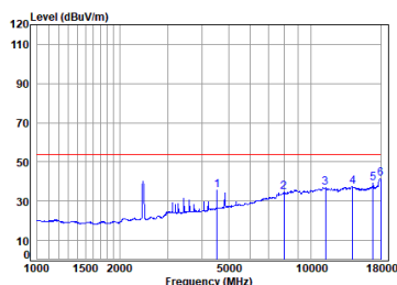
11ax_40M_TX_CH_06_Horizontal-Avg
