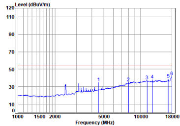
11n_HT(40M)_TX_CH_06_Vertical-Avg
