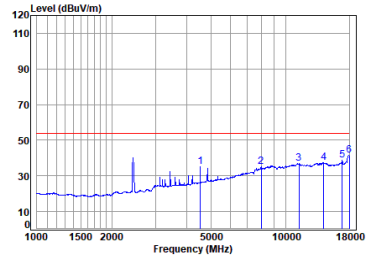
11n_HT(40M)_TX_CH_06_Horizontal-Avg
