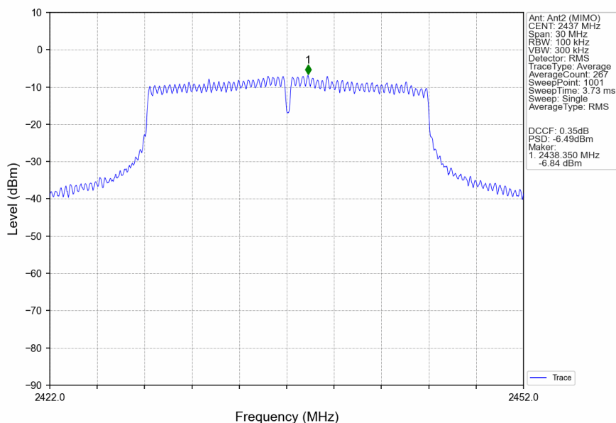
802.11ax(HEW20) MCH 2437MHz RU242 Left MIMO NTN
