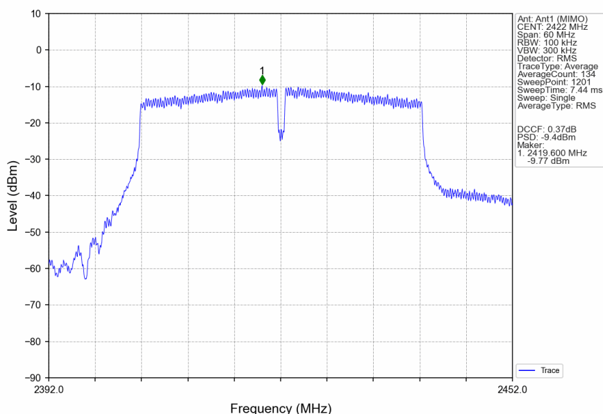
802.11n(HT40) LCH 2422MHz Ant1 (MIMO) NTN
