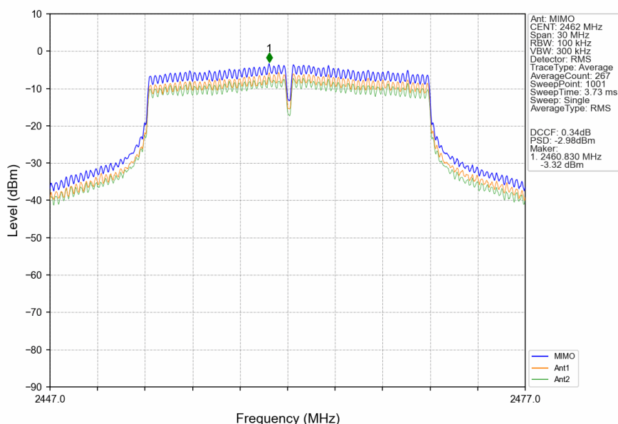
802.11ax(HEW20) HCH 2462MHz RU242 Left MIMO NTN
