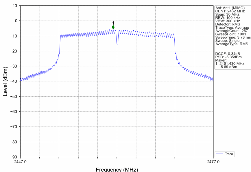
802.11ax(HEW20) HCH 2462MHz RU242 Left Ant1 (MIMO) NTN7
