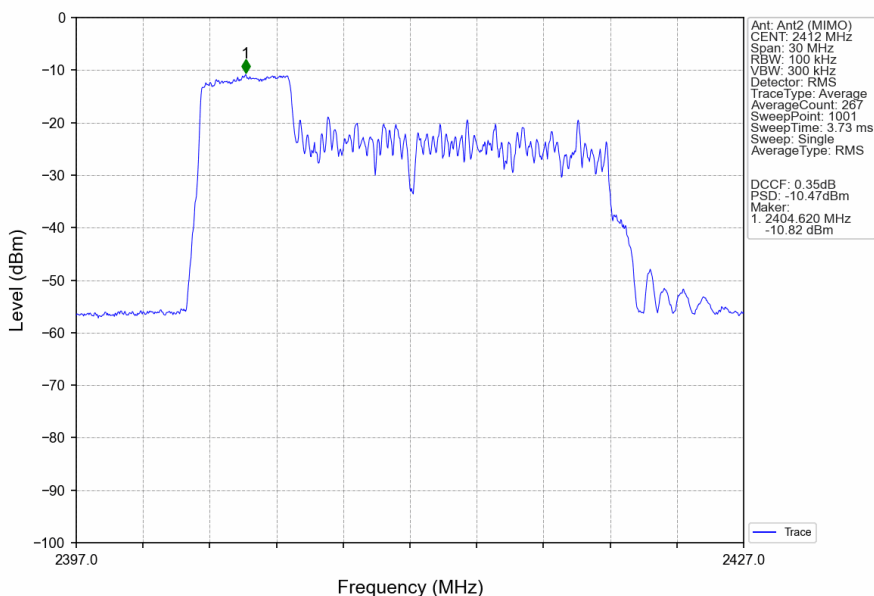
802.11ax(HEW20) LCH 2412MHz RU52 Left MIMO NTN
