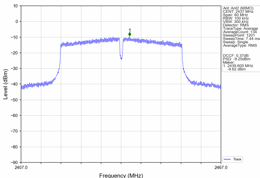
802.11n(HT40) MCH 2437MHz Ant2 (MIMO) NTV
