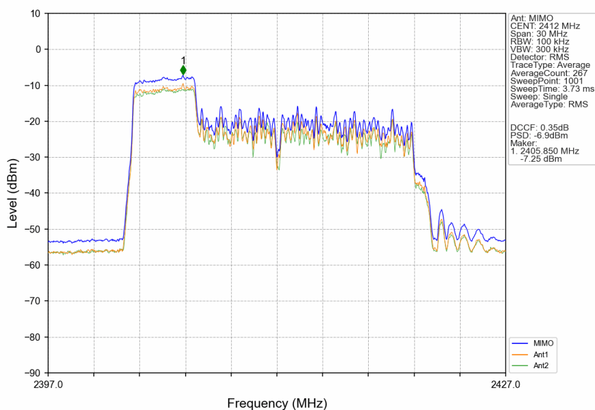
802.11ax(HEW20) LCH 2412MHz RU52 Left MIMO NTN
