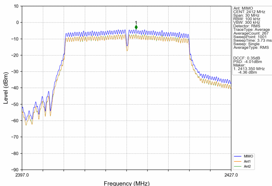
802.11ax(HEW20) LCH 2412MHz RU242 Left MIMO NTN
