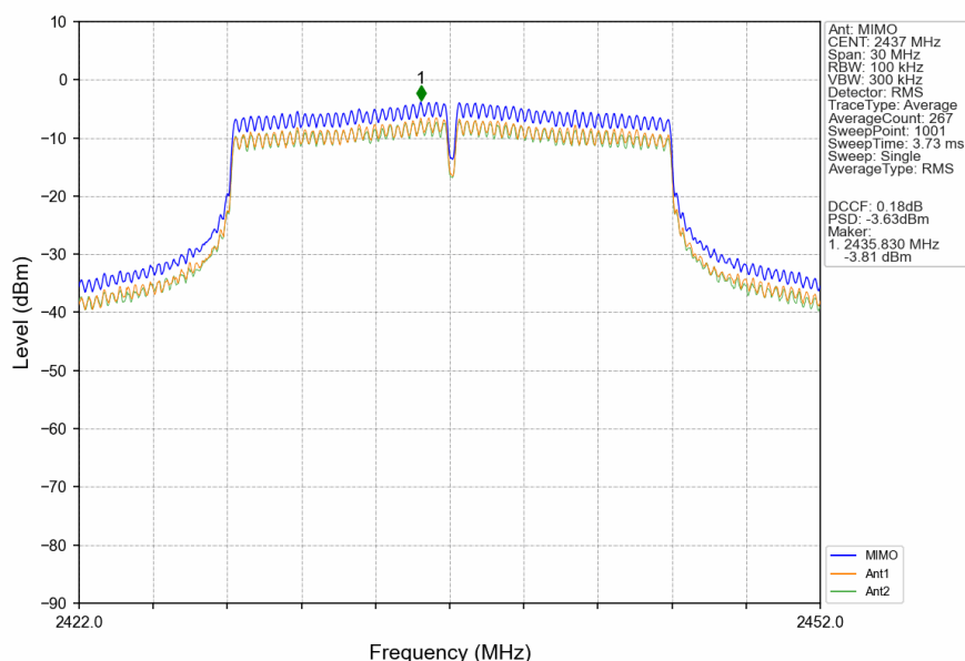
802.11n(HT20) MCH 2437MHz MIMO NTN
