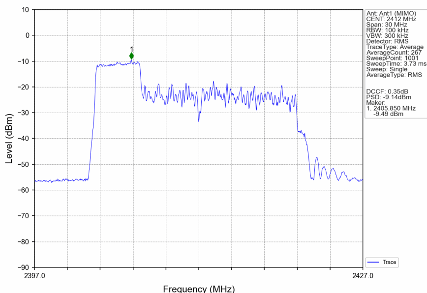
802.11ax(HEW20) LCH 2412MHz RU52 Left Ant1 (MIMO) NTN
