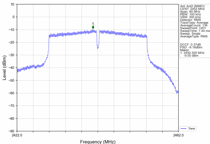
802.11n(HT40) HCH 2452MHz MIMO NTNV
