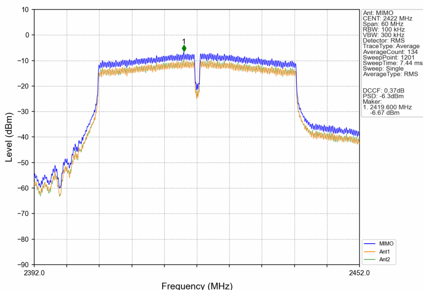
802.11n(HT40) LCH 2422MHz MIMO NTNV
