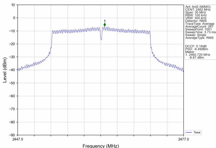
802.11n(HT20) HCH 2462MHz Ant2 (MIMO) NTNV
