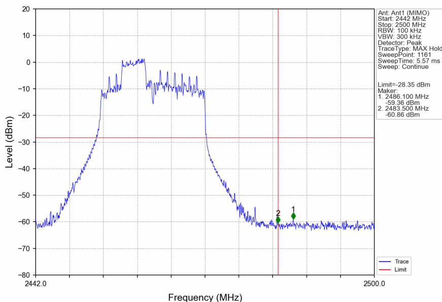
802.11ax(HEW20) HCH 2462MHz RU52 Right Ant1 (MIMO) NTNV
