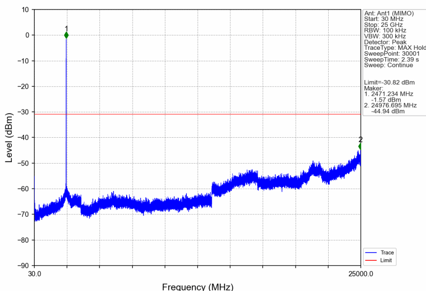
802.11ax(HEW20) HCH 2462MHz RU26 Right Ant1 (MIMO) NTNV
