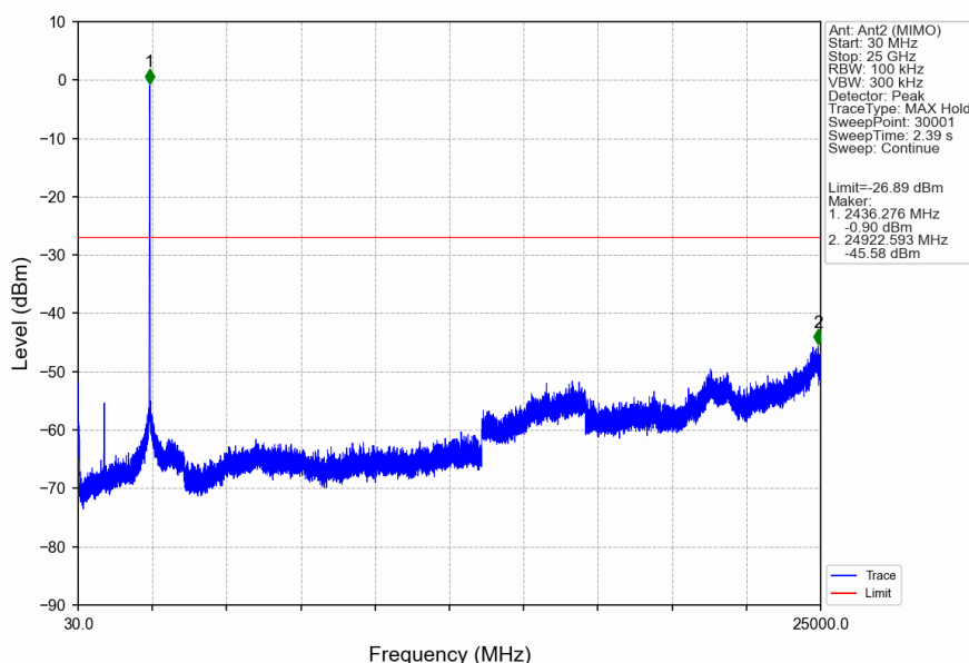
802.11ax(HEW20) MCH 2437MHz RU242 Left Ant2 (MIMO) NTV
