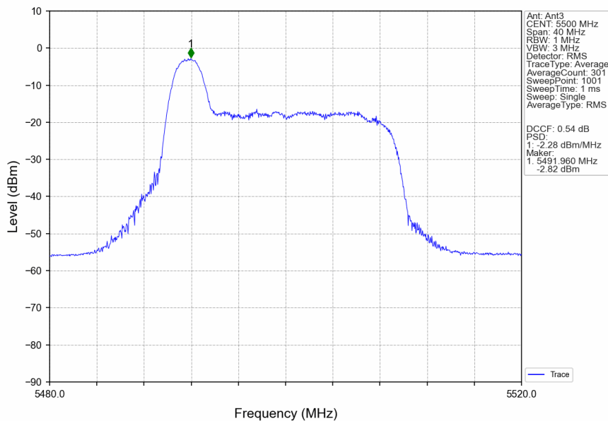
802.11ax(HEW20)_LCH_5500MHz_RU26_Left_Ant3_NTNV
