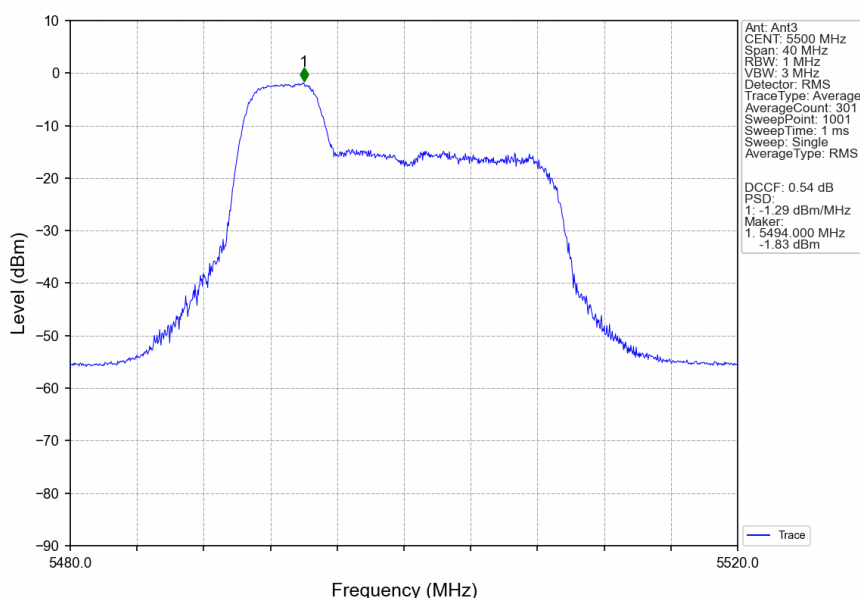
802.11ax(HEW20)_LCH_5500MHz_RU52_Left_Ant3_NTNV
