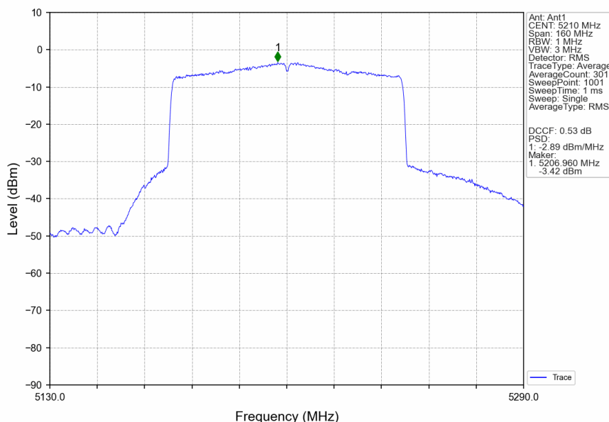
802.11ax(HEW80)_MCH_5210MHz_RU996_Left_Ant1_NTNV
