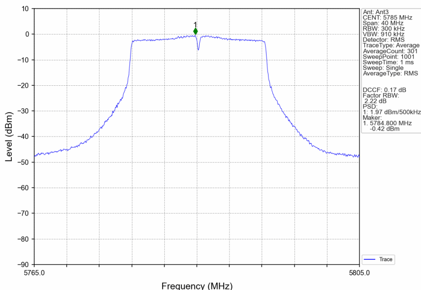
802.11a_MCH_5785MHz_Ant3_NTNV
