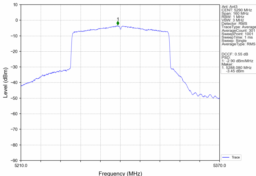
802.11ax(HEW80)_MCH_5290MHz_RU996_Left_Ant3_NTNV
