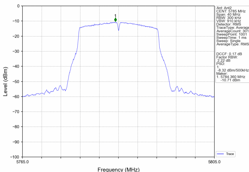
802.11a_MCH_5785MHz_Ant2_NTNV
