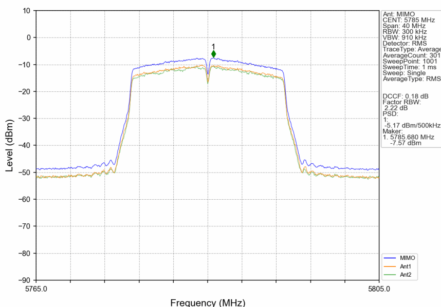
802.11n(HT20)_MCH_5785MHz_MIMO_NTNV
