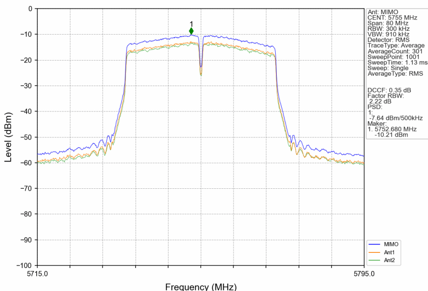
802.11n(HT40)_LCH_5755MHz_MIMO_NTNV
