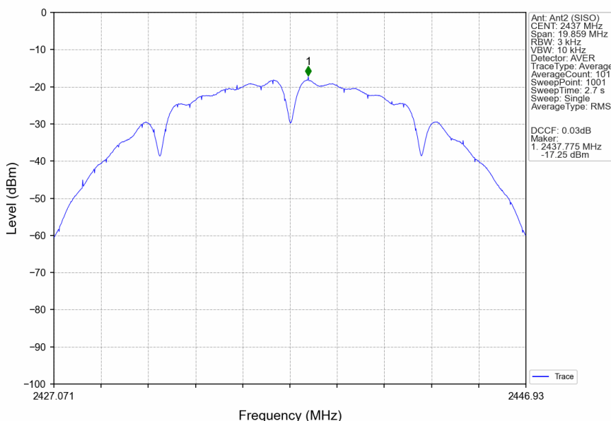
802.11b_MCH_2437MHz_Ant2 (SISO)_NTNV
