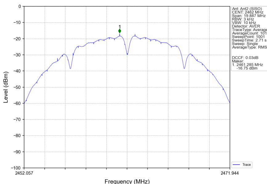
802.11b_HCH_2462MHz_Ant2 (SISO)_NTNV
