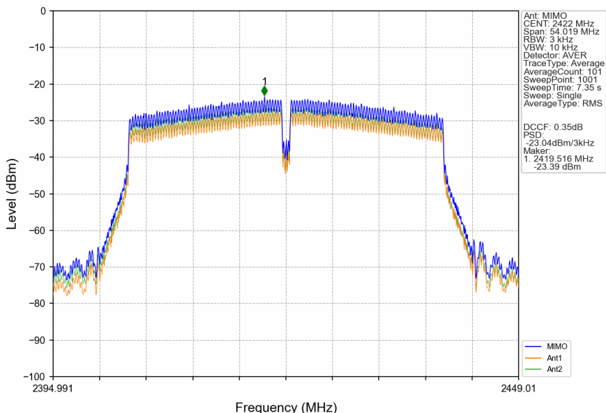
802.11n(HT40)_LCH_2422MHz_MIMO_NTNV
