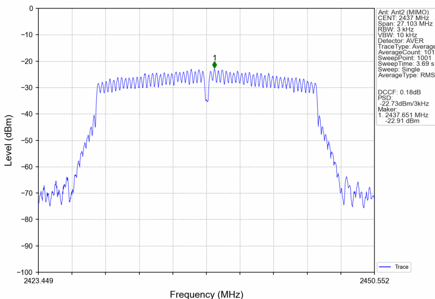
802.11n(HT20)_MCH_2437MHz_MIMO_NTNV
