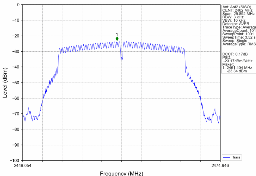
802.11g_HCH_2462MHz_Ant2 (SISO)_NTNV
