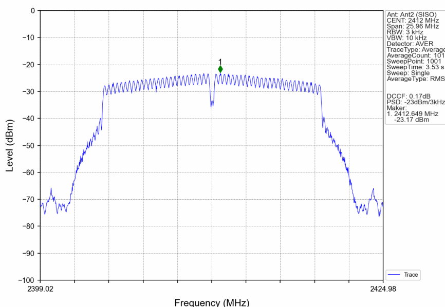
802.11g_LCH_2412MHz_Ant2 (SISO)_NTNV
