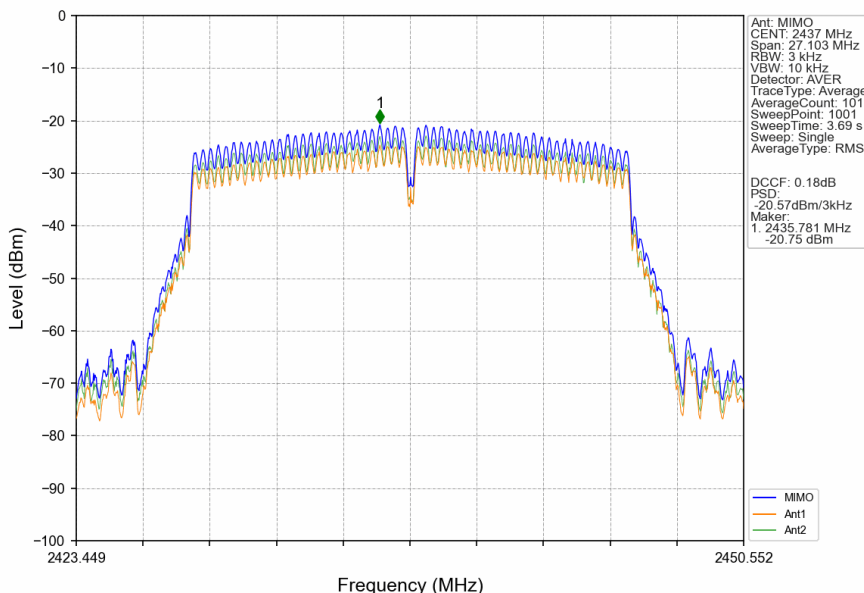
802.11n(HT20)_MCH_2437MHz_MIMO_NTNV
