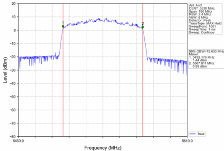
802.11ac(VHT80)_LCH_5530MHz_Ant1_NTNV
