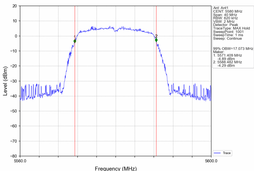
802.11a_MCH_5580MHz_Ant1_NTNV
