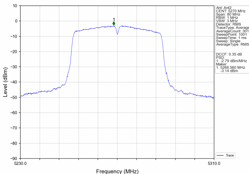
802.11n(HT40)_LCH_5270MHz_MIMO_NTNV
