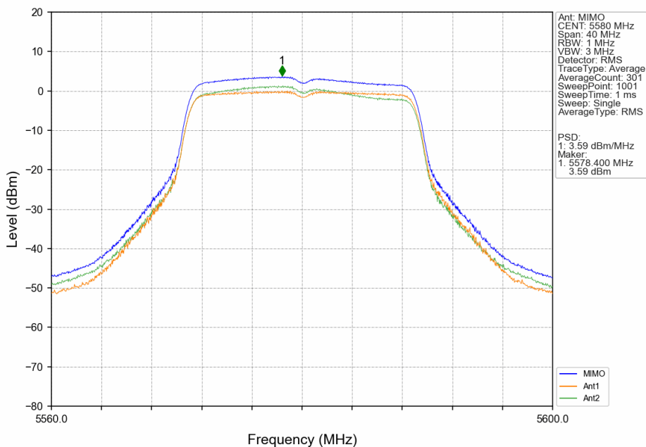
802.11n(HT20)_MCH_5580MHz_MIMO_NTNV
