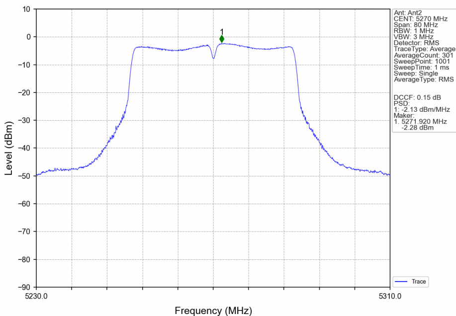
802.11n(HT40)_LCH_5270MHz_MIMO_NTNV
