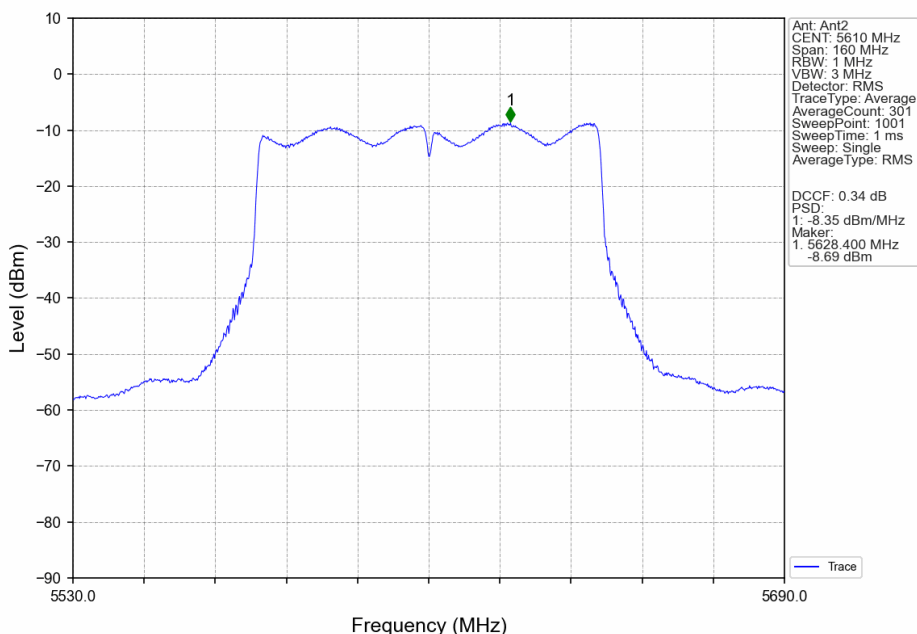
802.11ac(VHT80)_HCH_5610MHz_MIMO_NTNV
