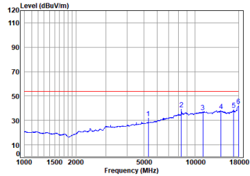
11n_HT(40M)_TX_CH_06_Horizontal-Avg
