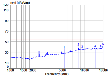
11n_HT(40M)_TX_CH_06_Vertical-Avg
