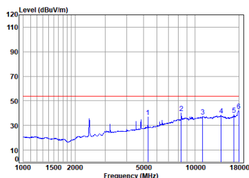
11n_HT(40M)_TX_CH_03_Vertical-Avg
