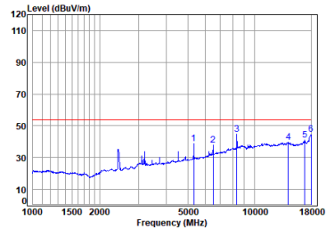
11ax_40M_TX_CH_06_Vertical-Avg
