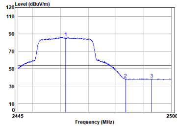
11ax_20M_TX_CH_11_Horizontal-Avg
