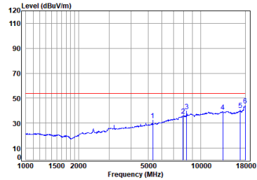
11ax_40M_TX_CH_06_Horizontal-Avg
