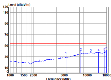
11n_HT(40M)_TX_CH_03_Horizontal-Avg
