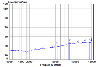
11n_HT(40M)_TX_CH_09_Horizontal-Avg
