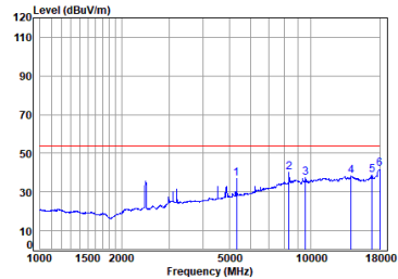
11n_HT(40M)_TX_CH_09_Vertical-Avg
