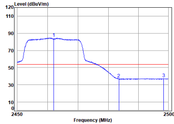
11n_HT(20M)_TX_CH_11_Horizontal-Avg
