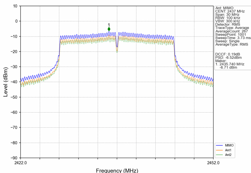
802.11n(HT20)_MCH_2437MHz_MIMO_NTNV
