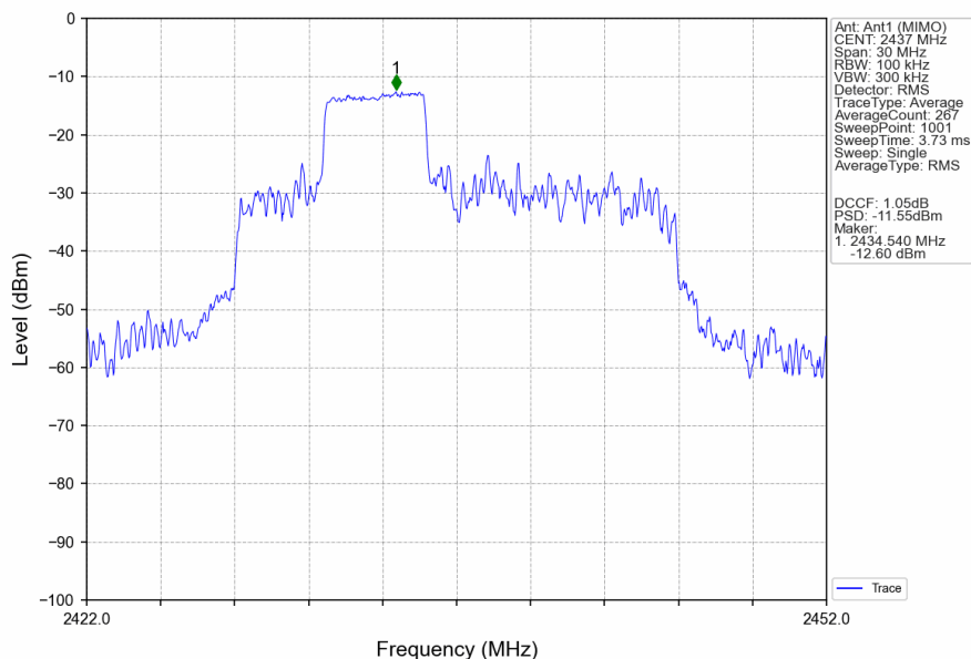
802.11ax(HEW20)_MCH_2437MHz_RU52_Mid_MIMO_NTNV
