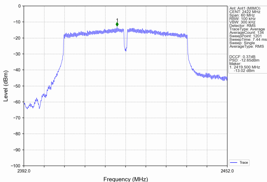
802.11n(HT40)_LCH_2422MHz_MIMO_NTNV
