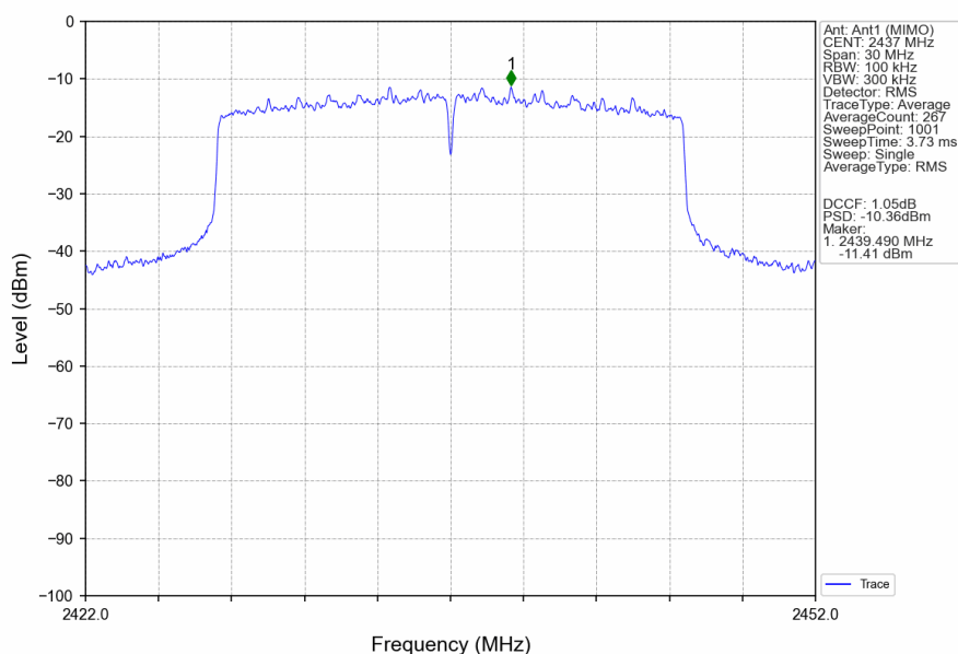
802.11ax(HEW20)_MCH_2437MHz_SU_/_MIMO_NTNV
