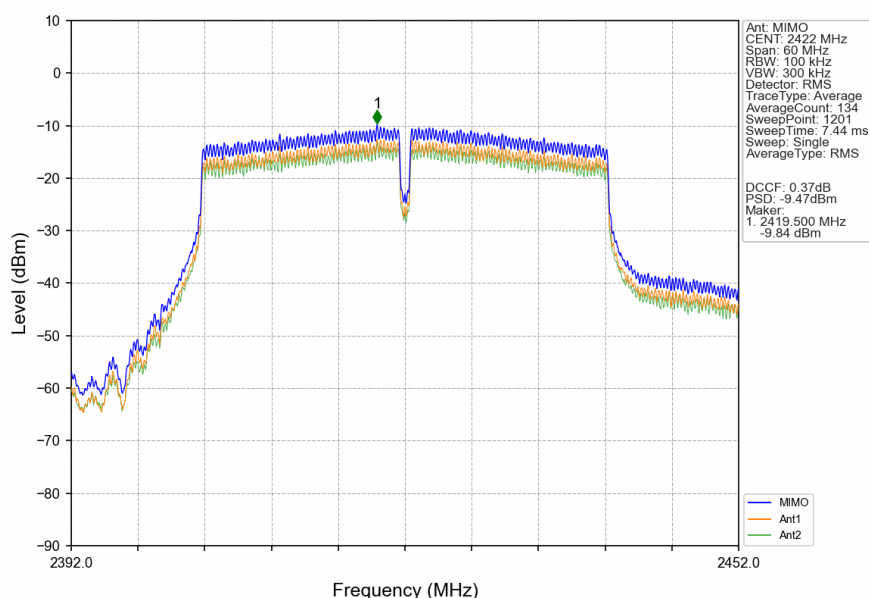
802.11n(HT40)_LCH_2422MHz_MIMO_NTNV
