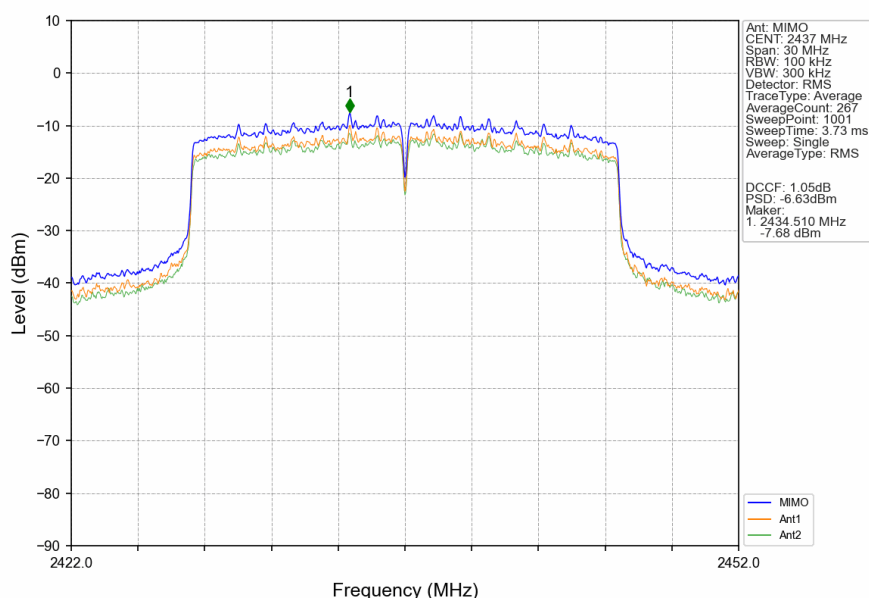
802.11ax(HEW20)_MCH_2437MHz_SU_/_MIMO_NTNV
