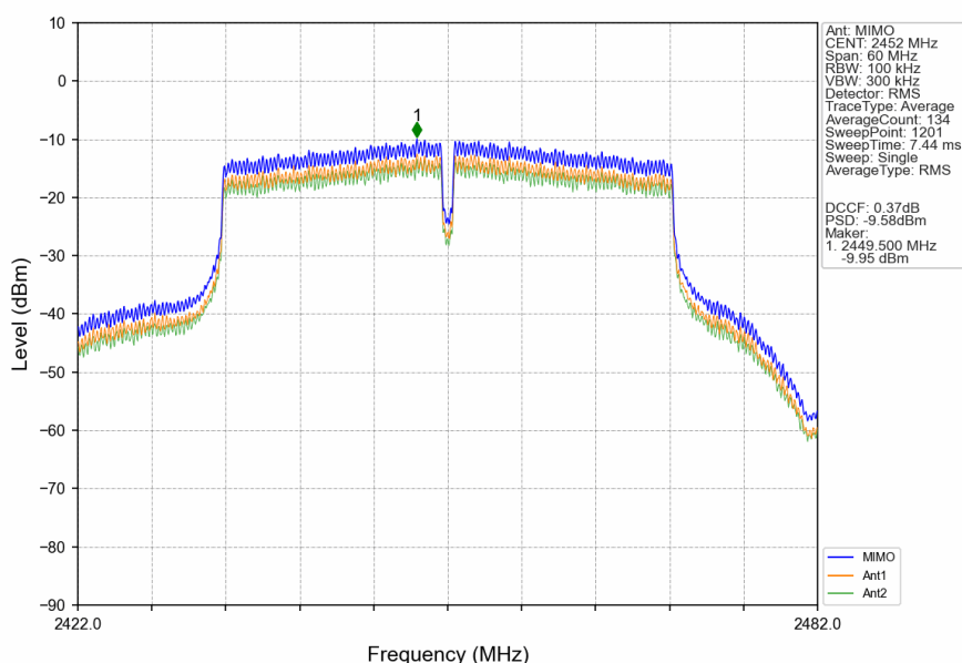
802.11n(HT40)_HCH_2452MHz_MIMO_NTNV
