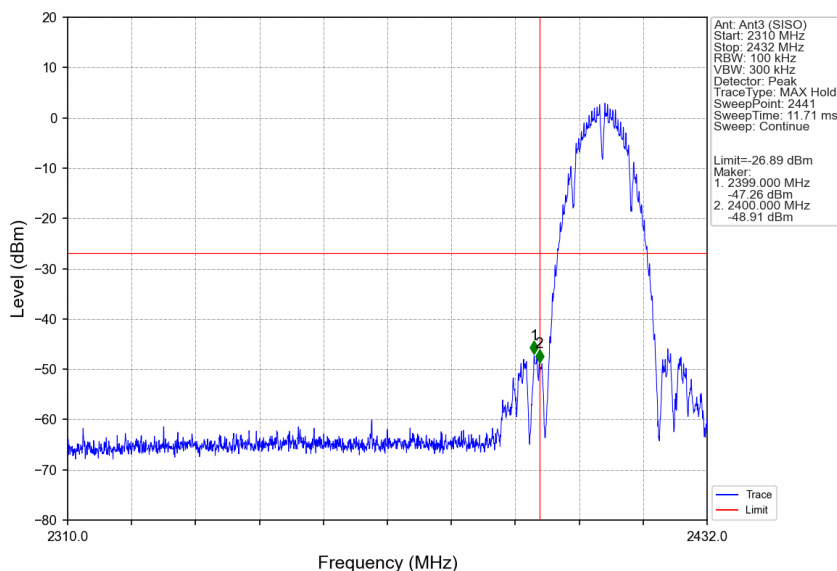
802.11b_LCH_2412MHz_Ant3 (SISO)_NTNV
