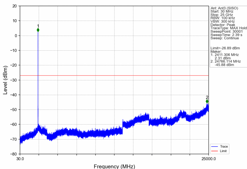
802.11b_LCH_2412MHz_Ant3 (SISO)_NTNV
