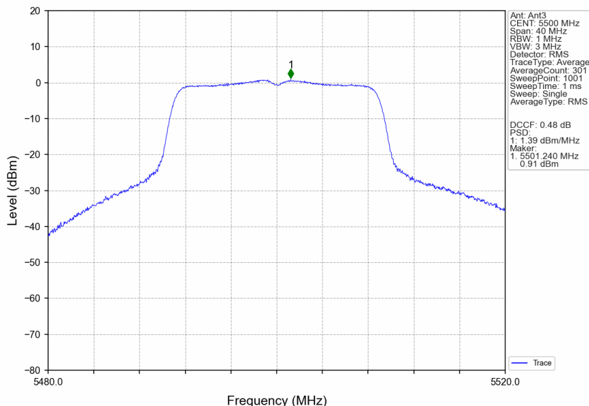
802.11ax(HEW20)_LCH_5500MHz_RU242_Left_Ant3_NTNV
