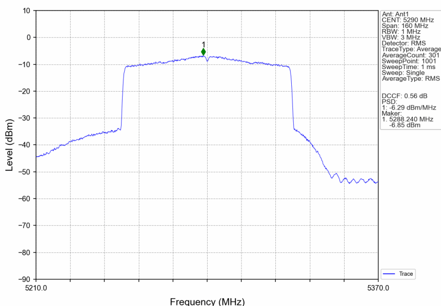
802.11ax(HEW80)_MCH_5290MHz_RU996_Left_Ant1_NTNV
