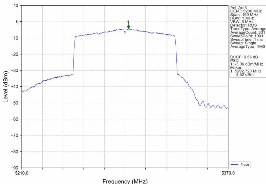
802.11ax(HEW80)_MCH_5290MHz_RU996_Left_Ant3_NTNV
