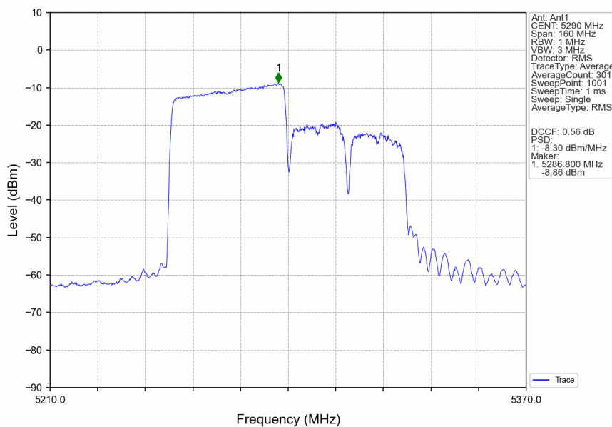
802.11ax(HEW80)_MCH_5290MHz_RU484_Left_Ant1_NTNV
