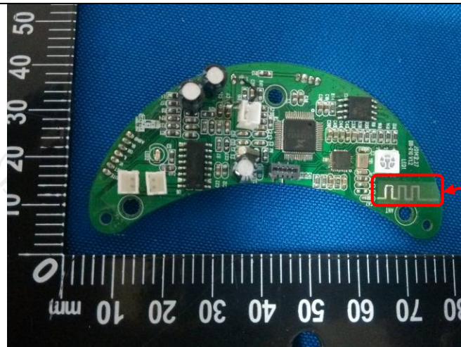
Antenna
