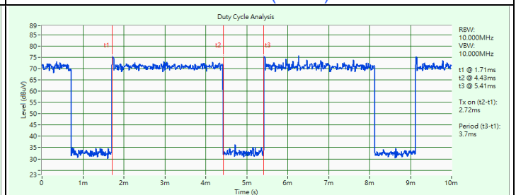
802.11ax (HE20) 52-tone RU
