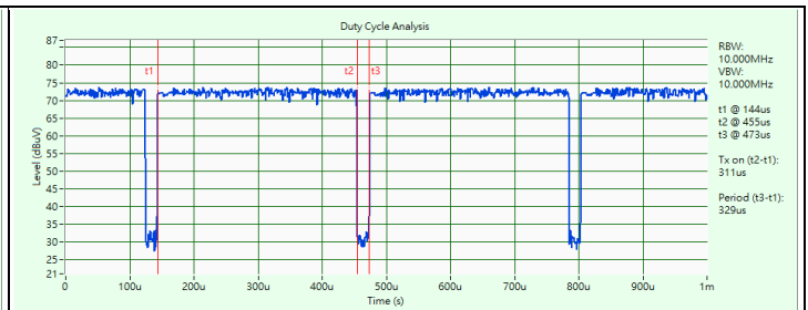
802.11ax (HE20)
