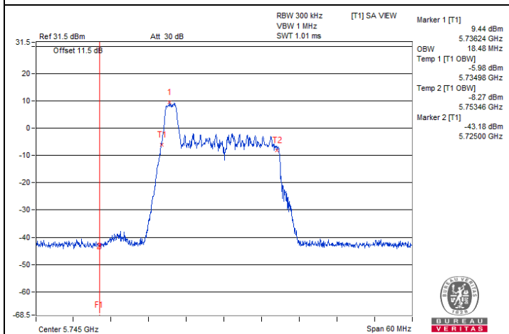
802.11ax (HE20) 26-tone RU: CH 149
