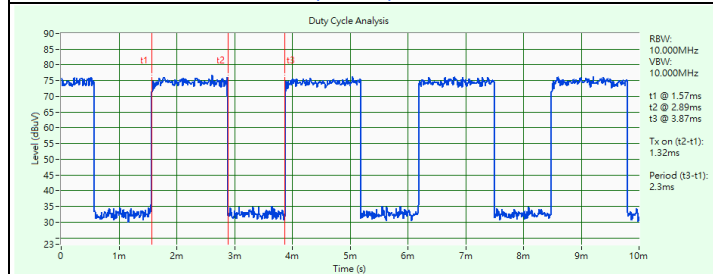
802.11ax (HE20) 106-tone RU
