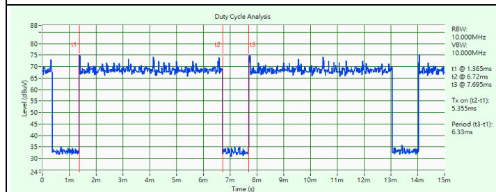
802.11ax (HE20) 26-tone RU
