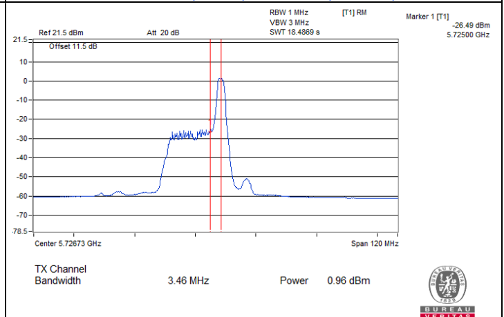
802.11ax (HE20) 26-tone RU: CH 144 (U-NII-3)
