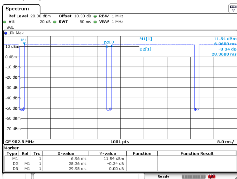
LoRa(DTS)SF 7
