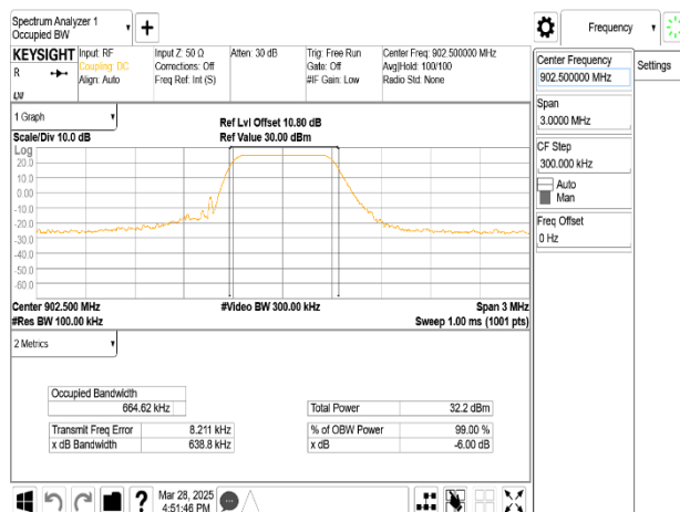
OBW_LoRa_SF11_LowCH-902.5MHz
