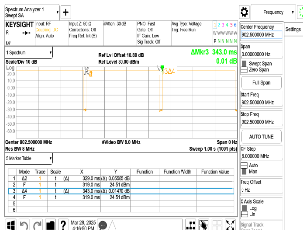
LoRa_SF11_LowCH-902.5MHz
