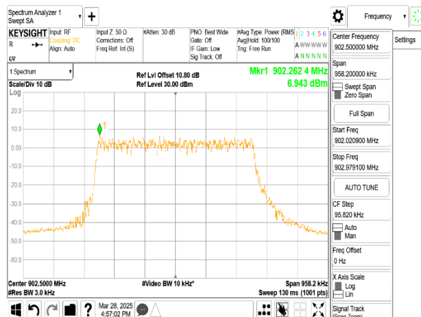
PSD_LoRa_SF11_LowCH-902.5MHz
