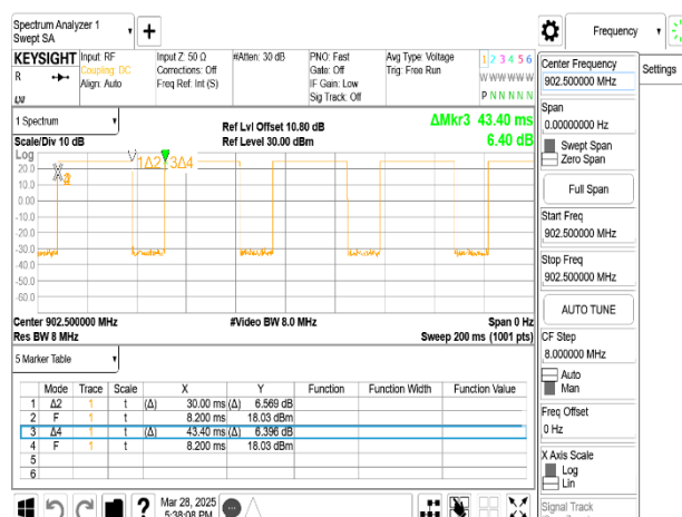
LoRa_SF7_LowCH-902.5MHz
