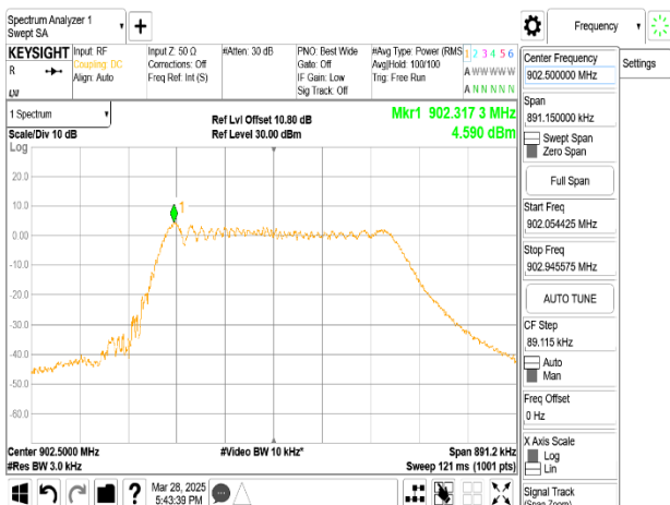
PSD_LoRa_SF7_LowCH-902.5MHz
