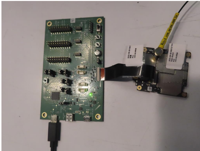
EUT
