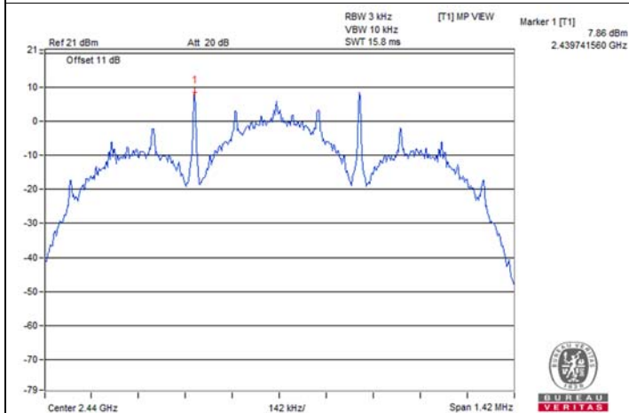
BT-LE 125k : CH 19
