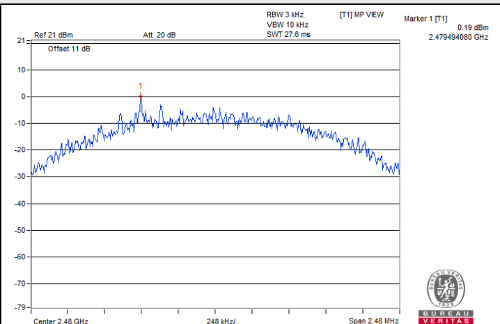
BT-LE 2M : CH 39
