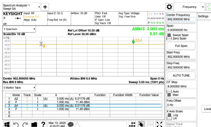
FSK 100Kbps 249bytes_LowCH-902.9MHz
