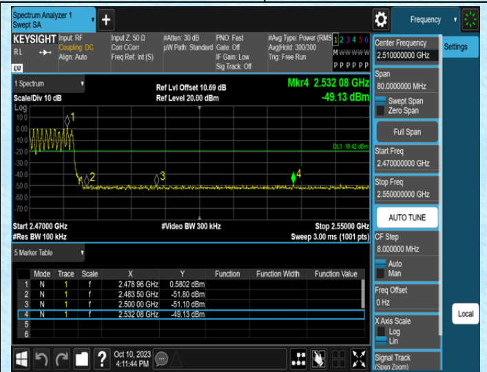
DH5-Ant1-Hop_2480
