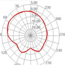
2450.000MHz E2
