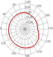
2400.000MHz E2
