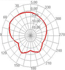
2450.000MHz H
