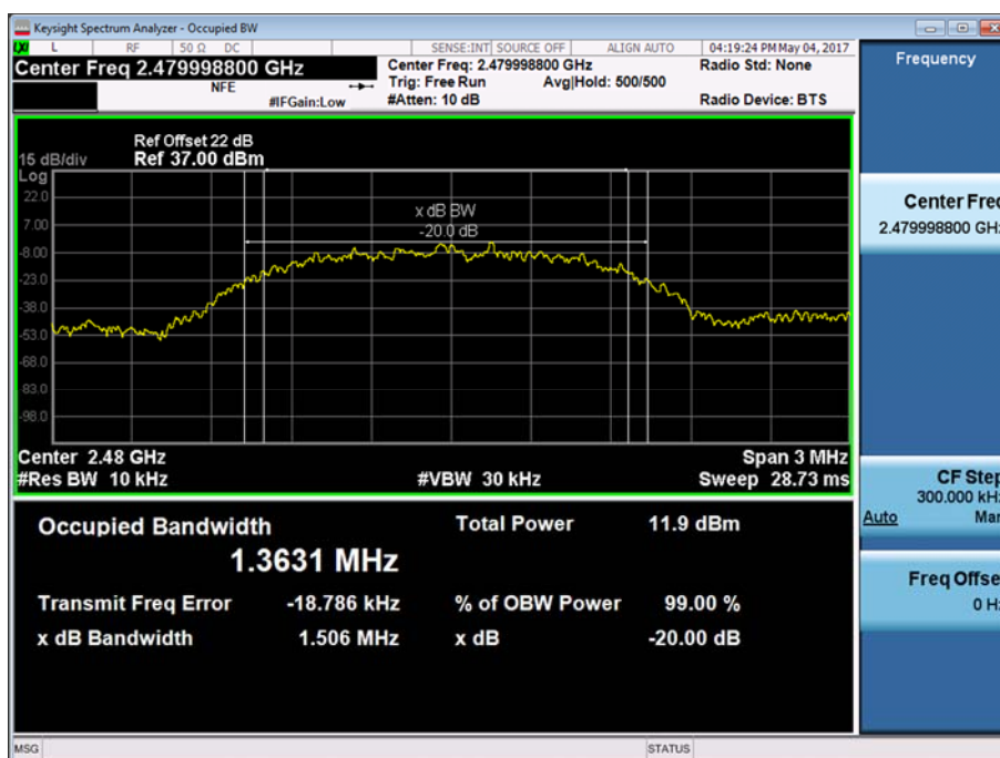
Figure 9 - 2480 MHz - \pi/4 DQPSK
