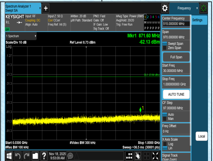
11G-Ant1-2437-30~1000-PASS
