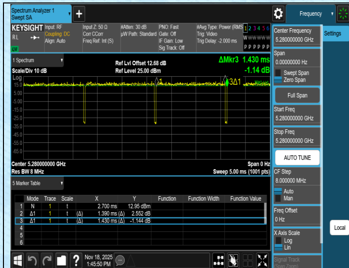
NTNV-11A-Ant1-5280
