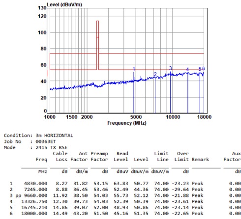
2.4G_SRD_LOW_TX_Horizontal
