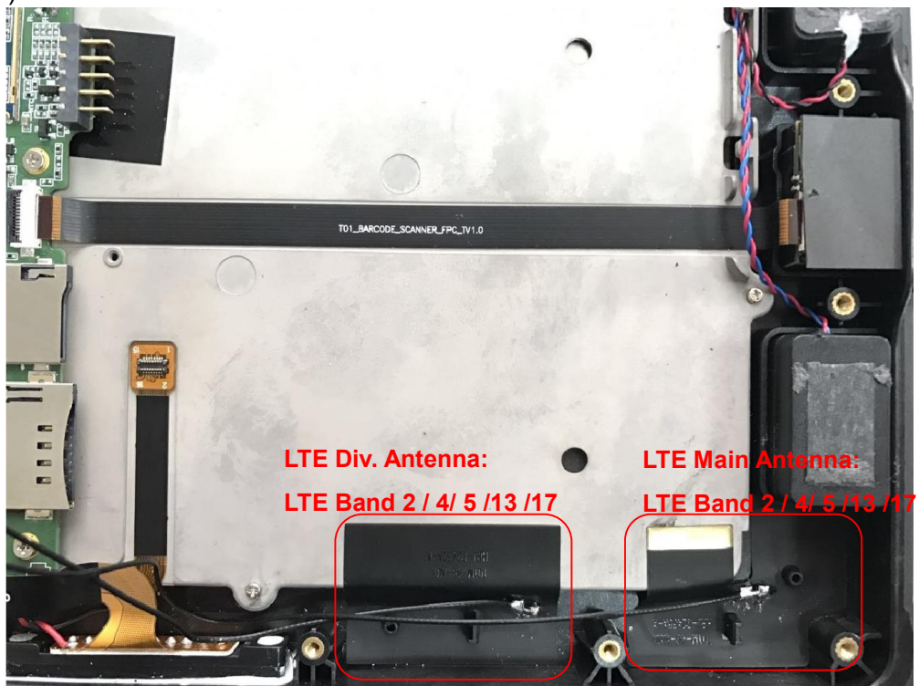
(24) EUT Photo
