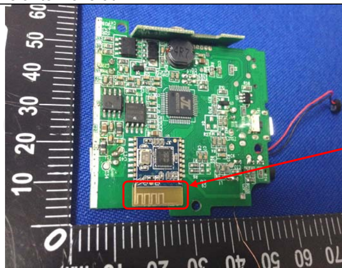
Antenna
