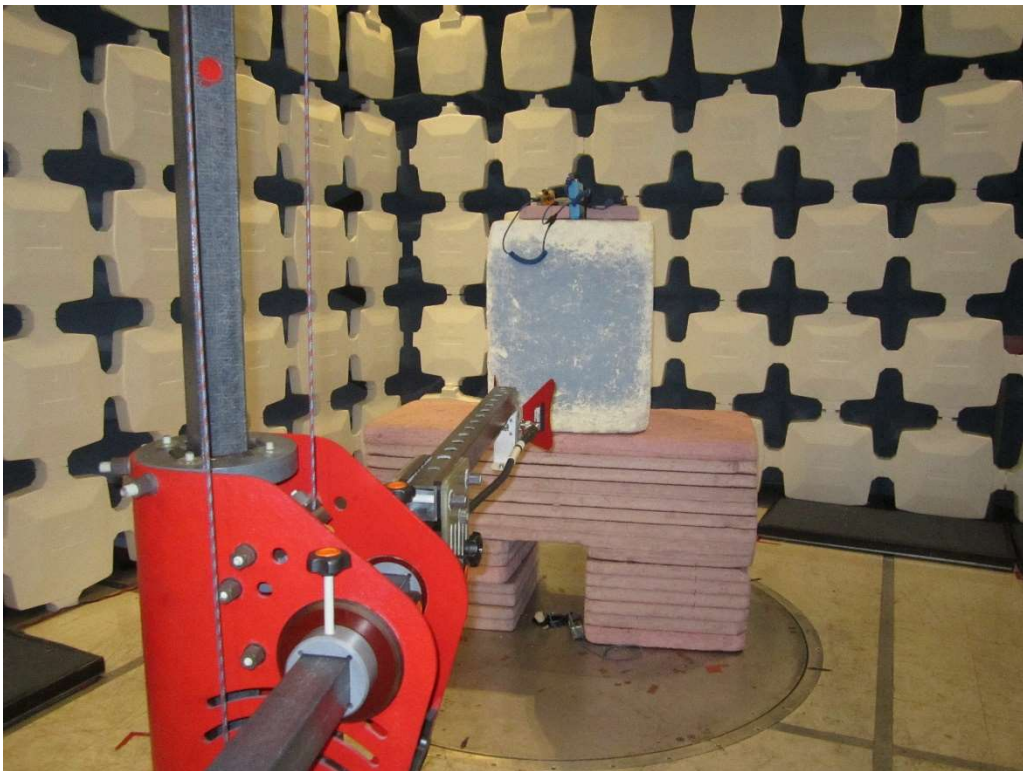
6GHz-10GHz
