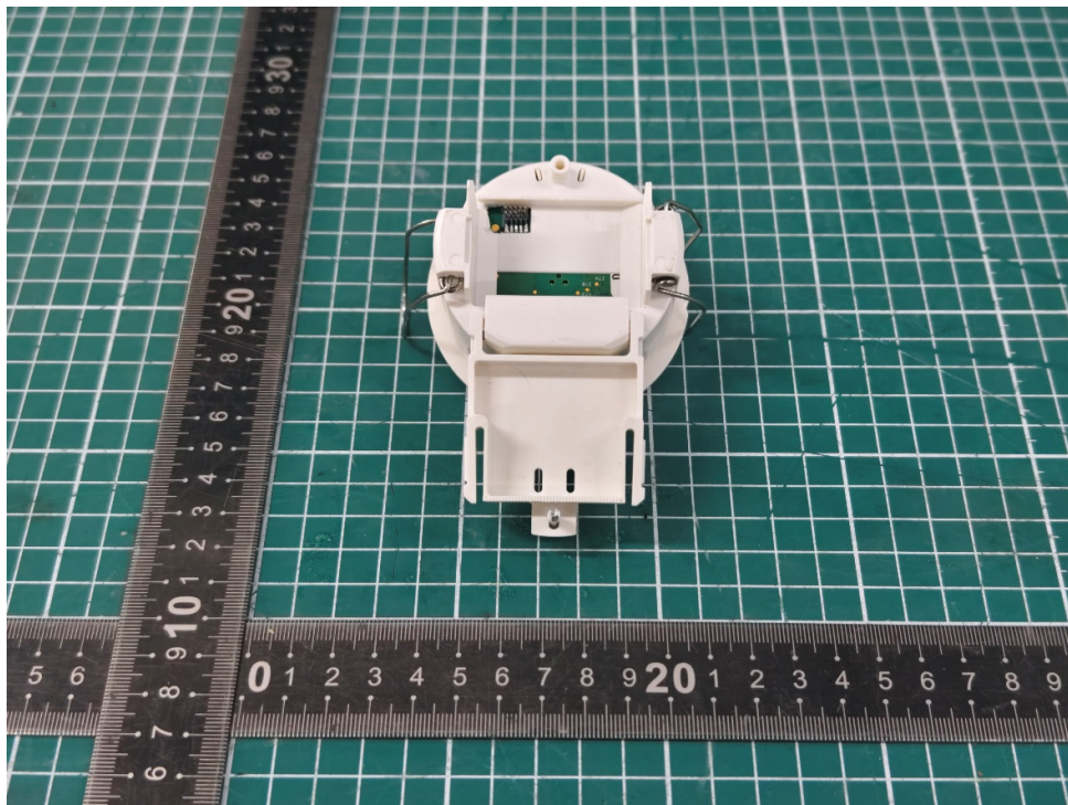
DNS360LB-CR-PIR-DyNet
