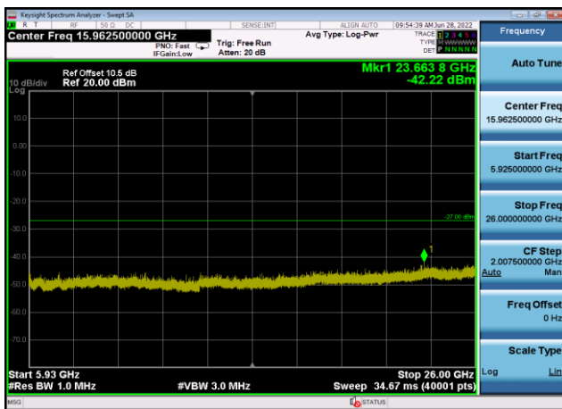
U-NII-3 ,Plot 3,5925MHz~26000MHz-802. 11ac(20MHz),5785MHz,Ant1
