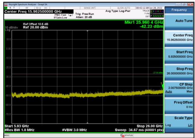
U-NII-3 ,Plot 3,5925MHz~26000MHz-802. 11ac(20MHz),5745MHz,Ant1
