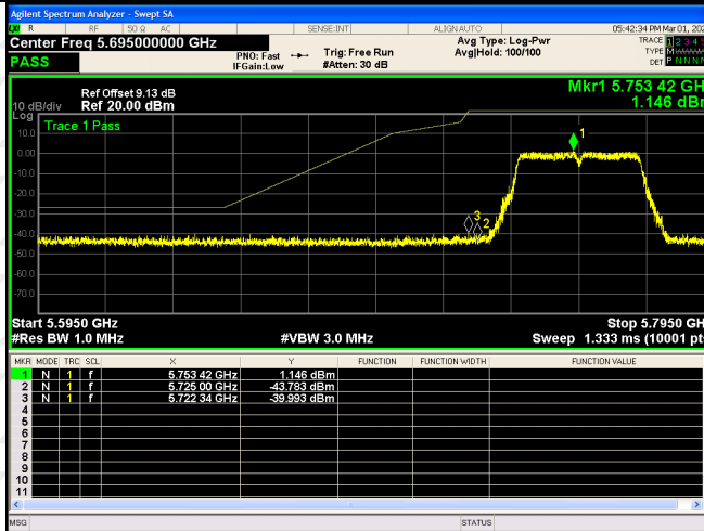
802.11ac(VH80)-5775
