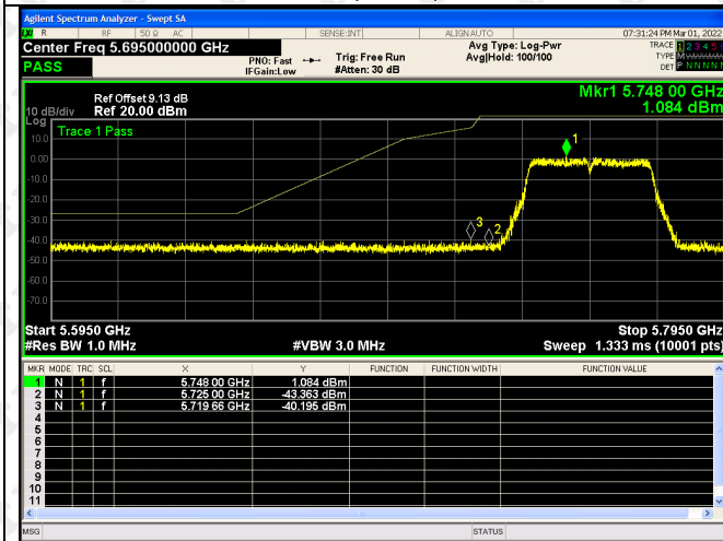
802.11ac(VH80)-5755
