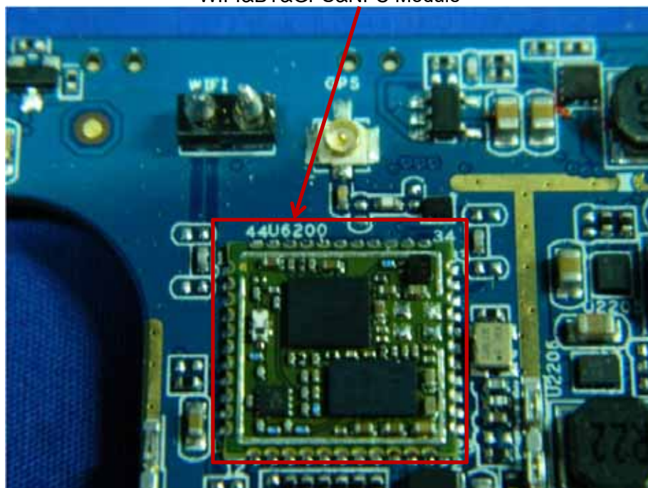
WIFI&BT&GPS&NFC Module
