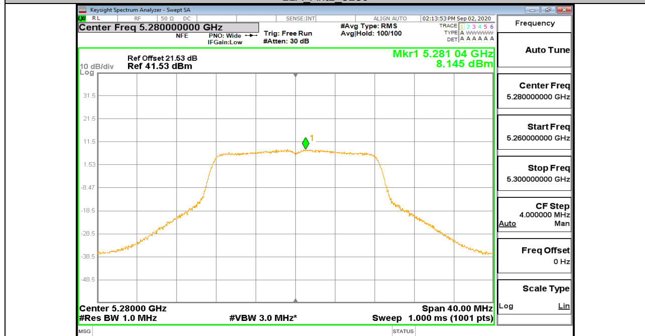
11A_Ant2_5280
