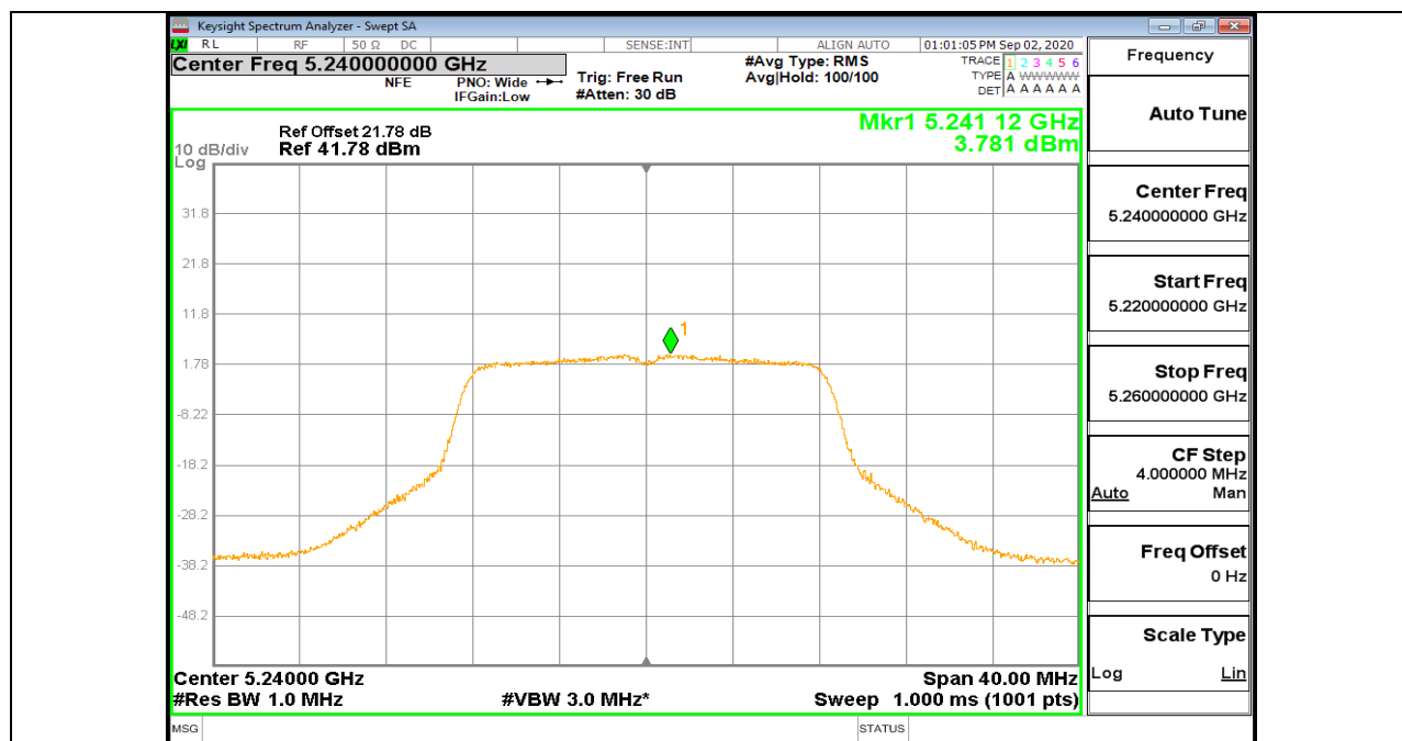
11A_Ant1_5240
