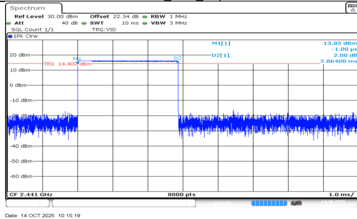
DH5_Ant2_Hop
