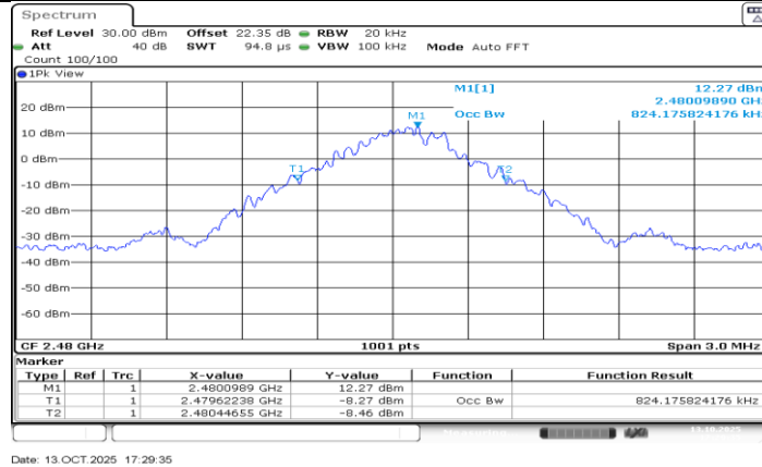
DH5_Ant2_2480
