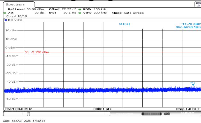
3DH5_Ant2_2480_30~1000
