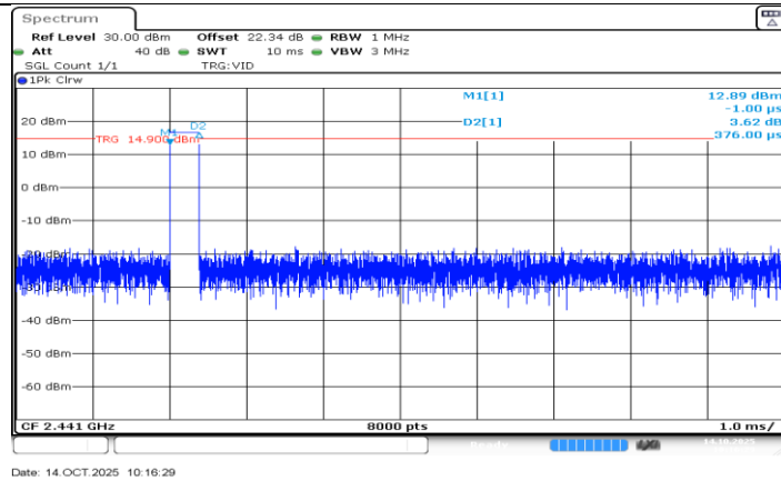
DH1_Ant2_Hop
