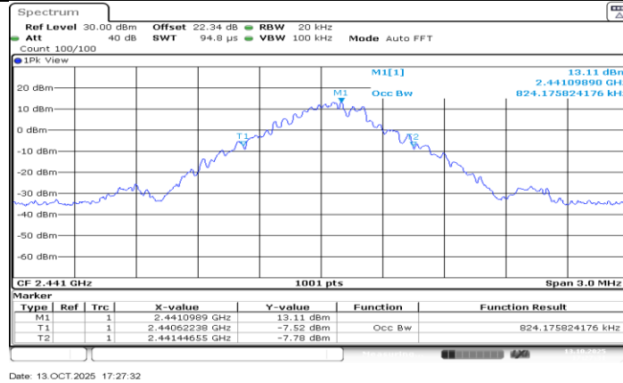
DH5_Ant2_2441
