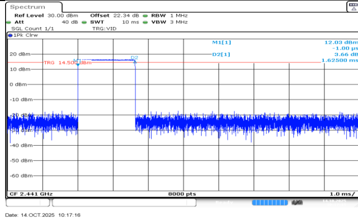
DH3_Ant2_Hop
