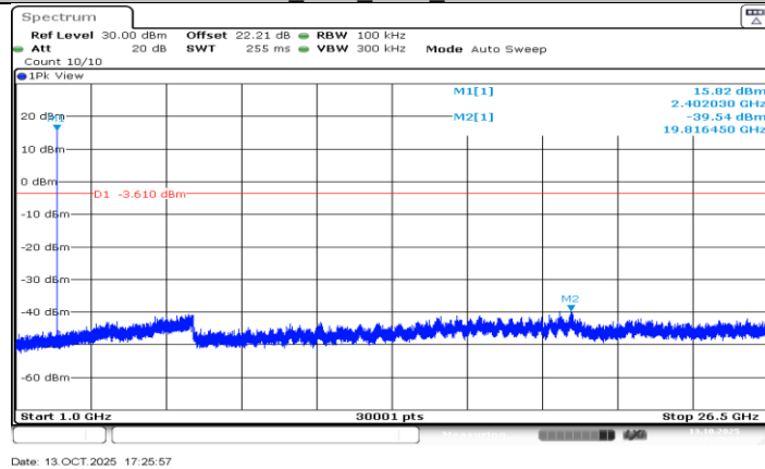
DH5_Ant2_2402_1000~26500
