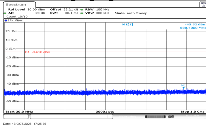
DH5_Ant2_2402_30~1000
