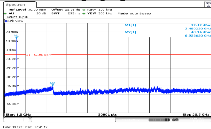
3DH5_Ant2_2480_1000~26500
