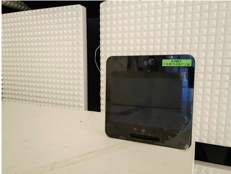
RADIATED SETUP (Z axis)
