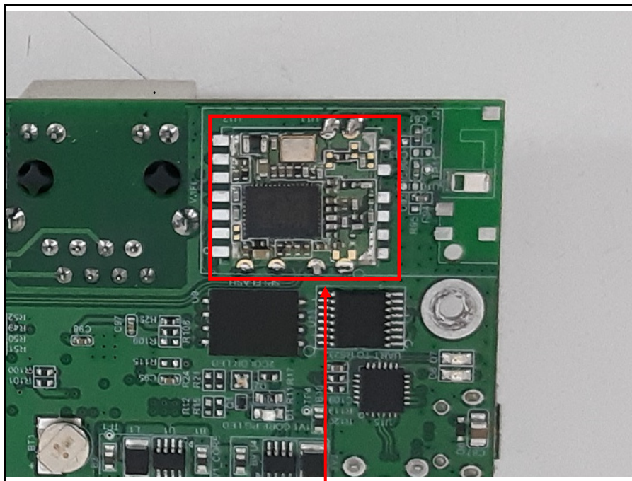
Wifi Module
