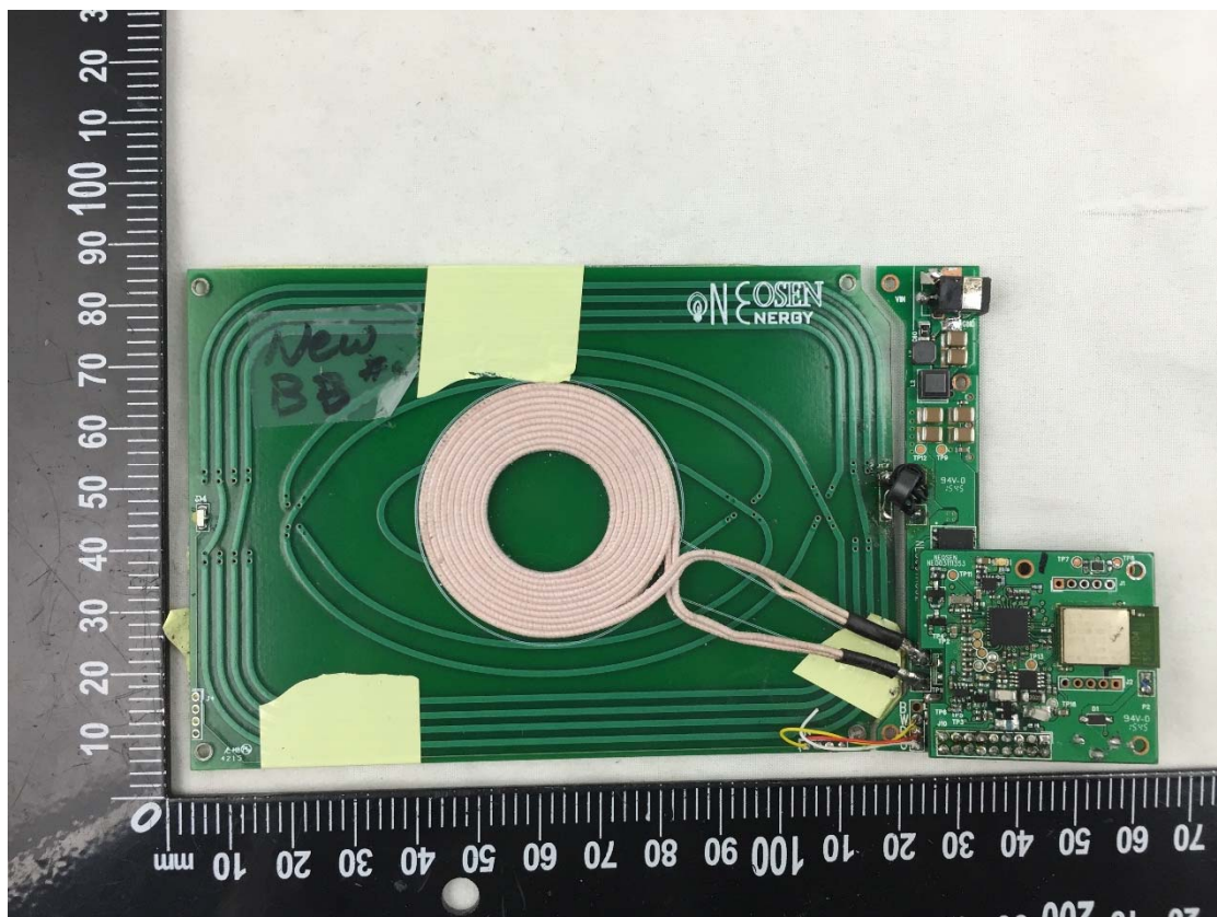
EUT Photo 4
