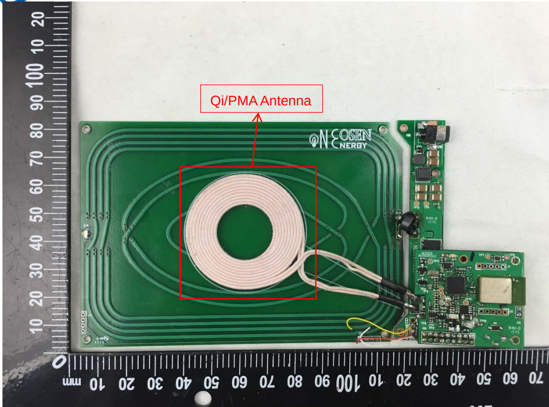
EUT Photo 5
