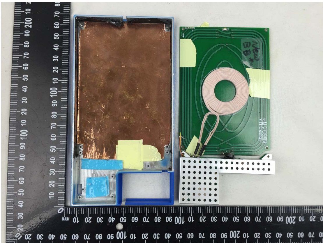
EUT Photo 2
