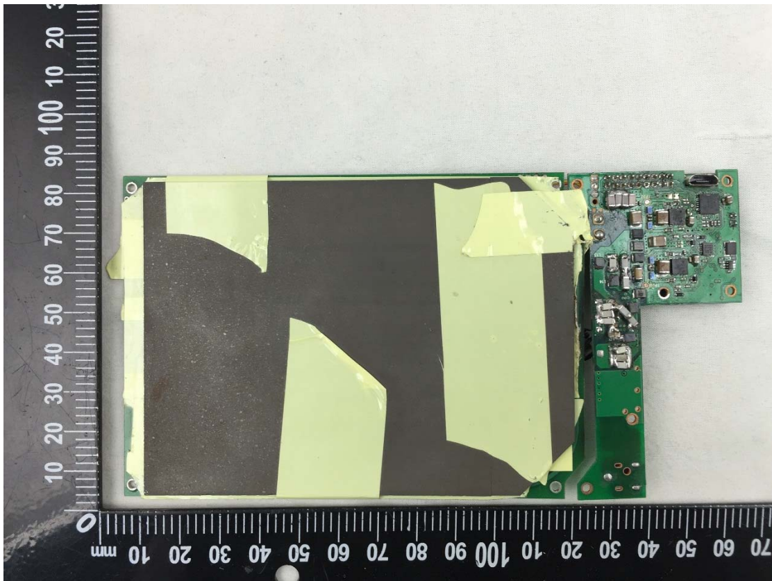
EUT Photo 3
