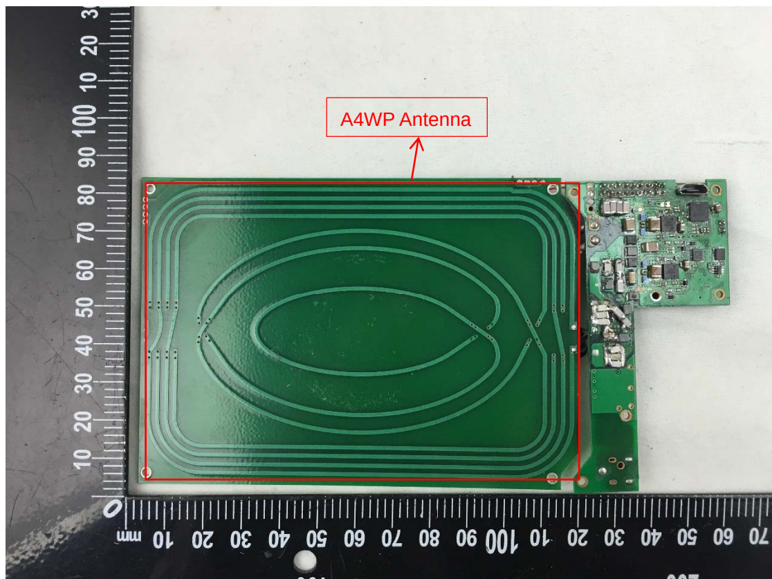
EUT Photo 6
