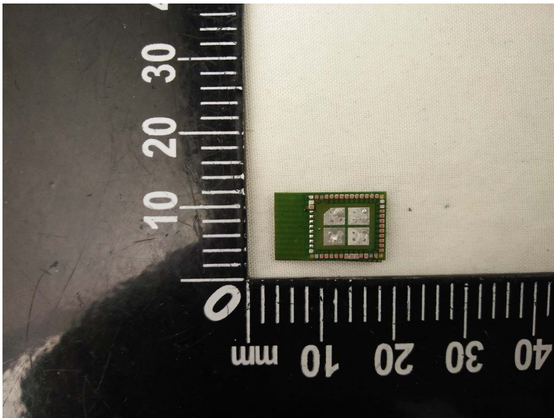
EUT Photo 10
