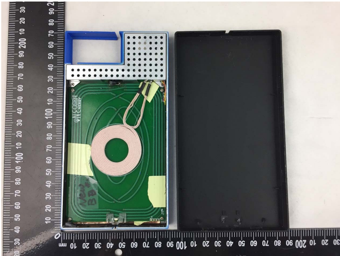
EUT Photo 1
