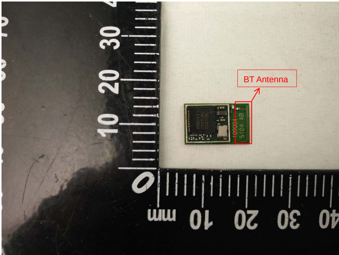
EUT Photo 11
