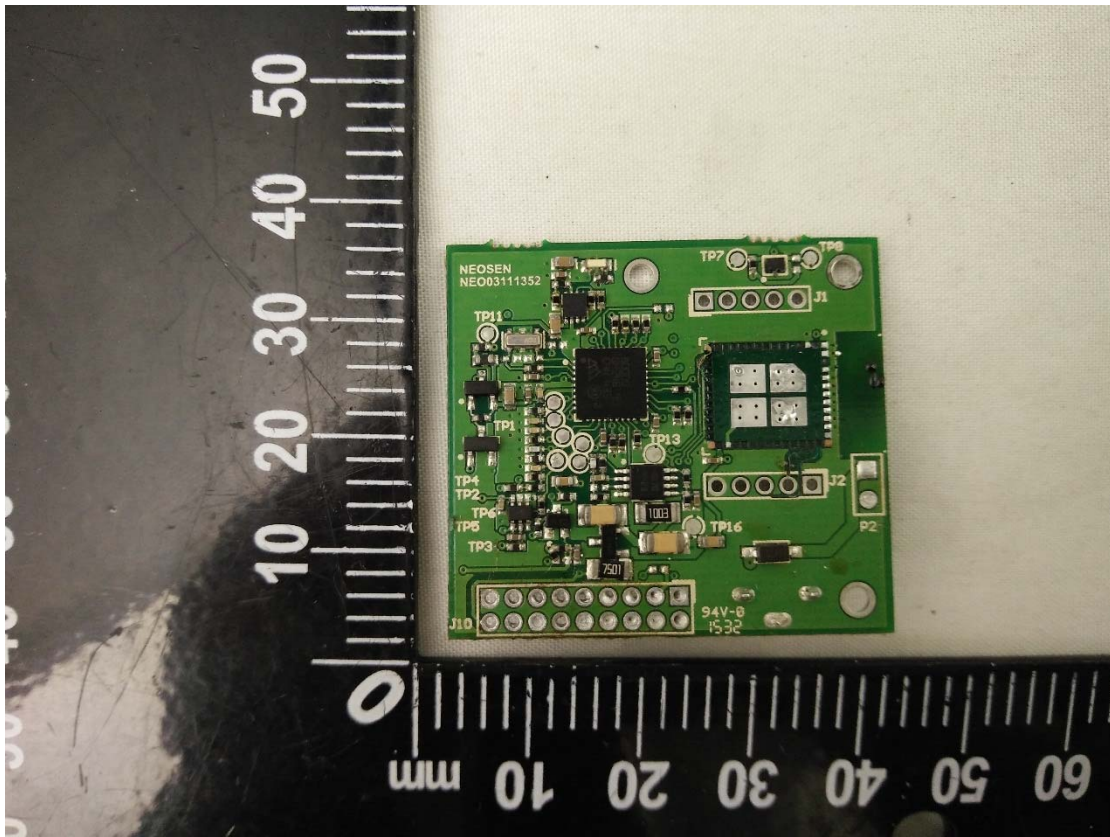
EUT Photo 9
