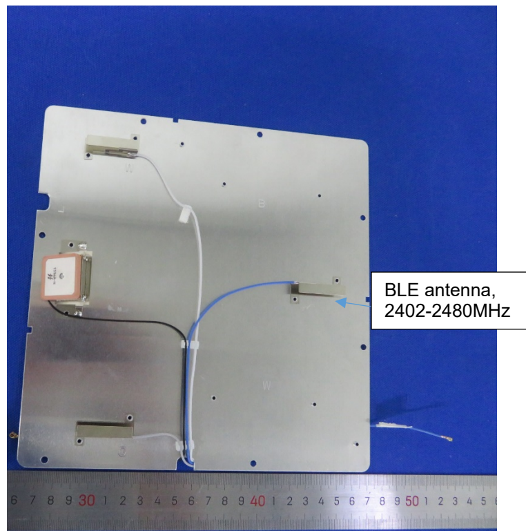
Antenna SA04WEG01RA
