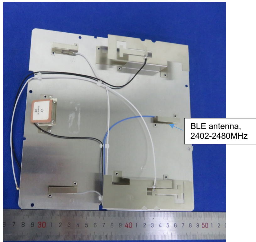
Antenna SA04WEG01RA
