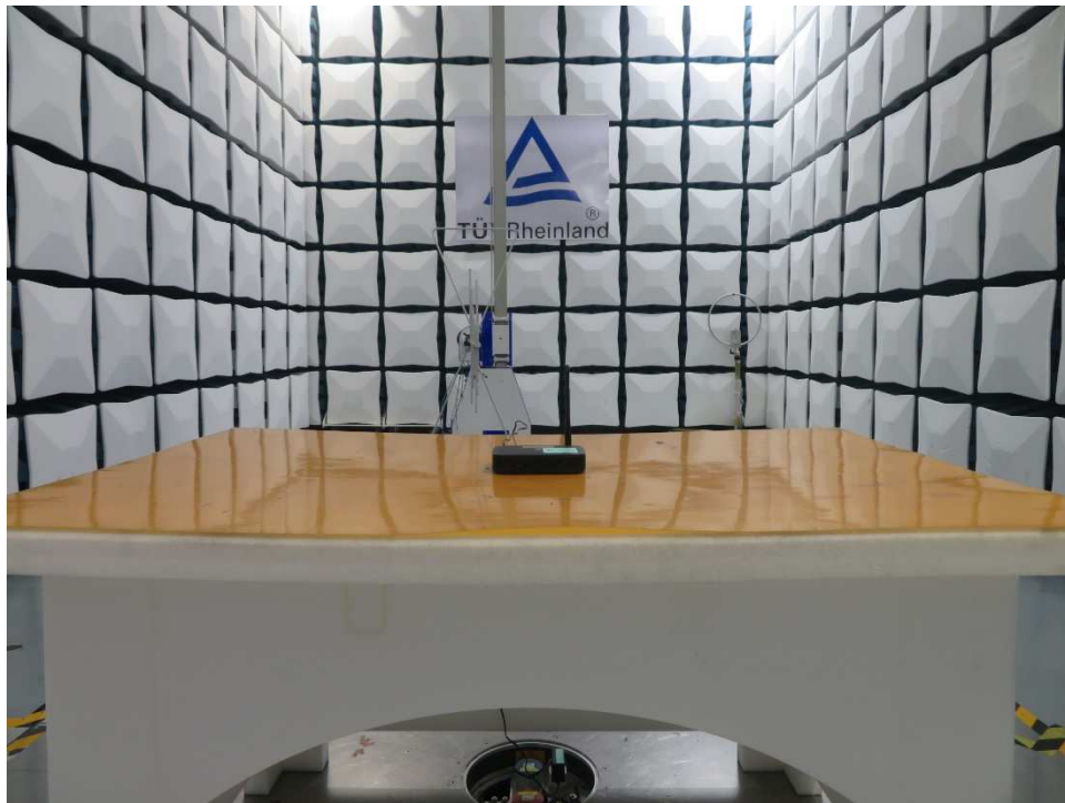
(Build-in LTE antenna)
