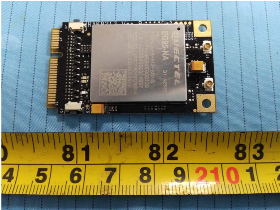
LTE module
